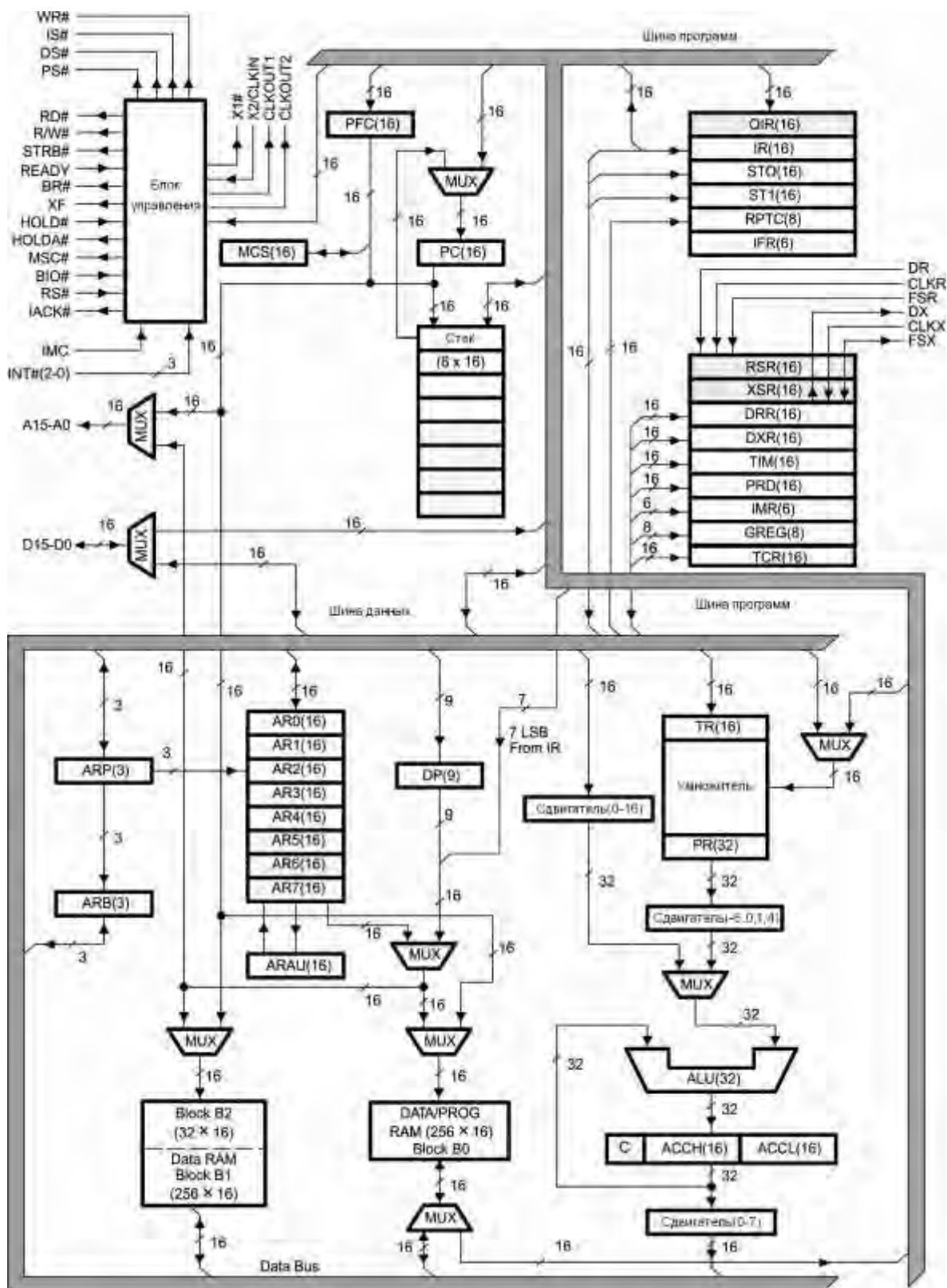
Рисунок 1, лист 1 – Схема электрическая структурная ИС 1867ВМ7Т
