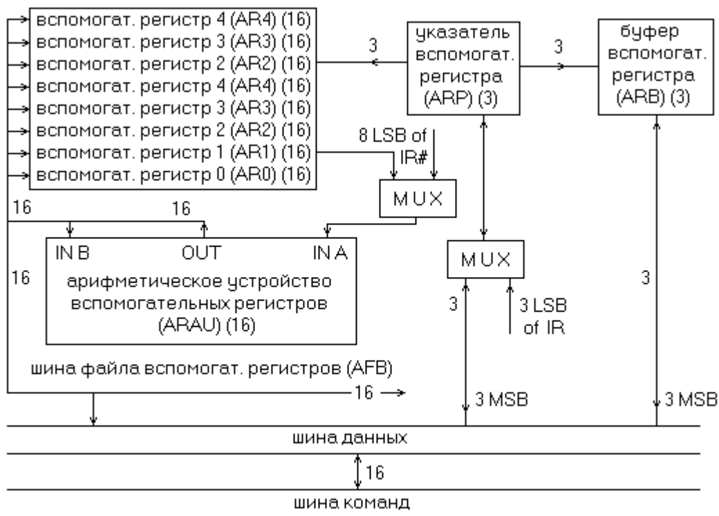
Рисунок 8 - Файл вспомогательных регистров
