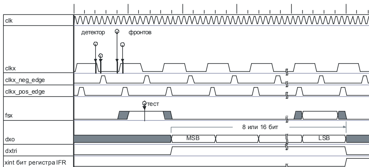
Рисунок 29 - Временная диаграмма передачи данных
