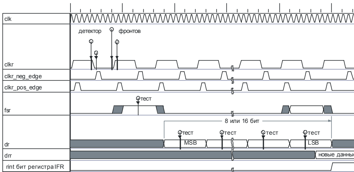
Рисунок 30 - Временная диаграмма приема данных
