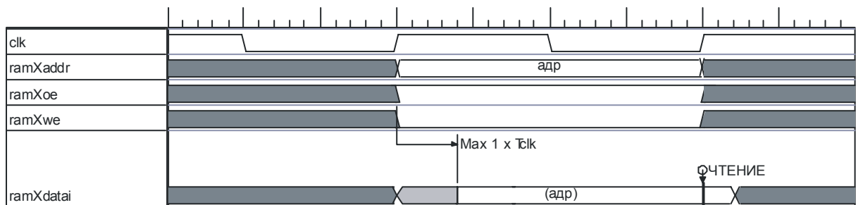
Рисунок 21 - Временная диаграмма режима прямого доступа к памяти Внутреннее ОЗУ – чтение
