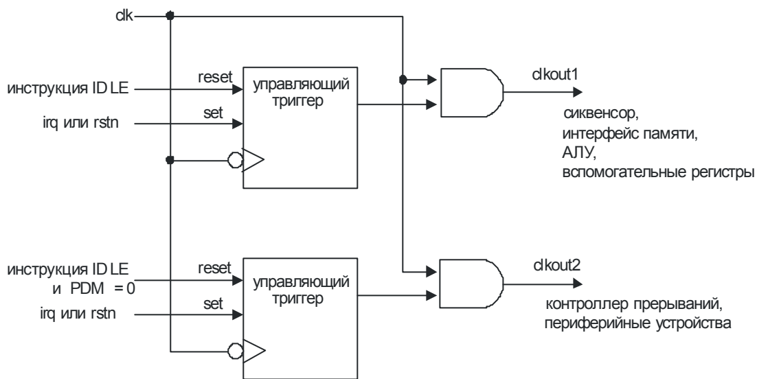
Рисунок 35 - Управление тактовыми сигналами
