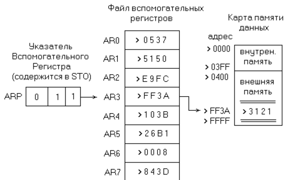
Рисунок 7 - Пример косвенной адресации с помощью вспомогательных регистров
