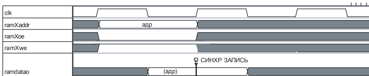
Рисунок 23 - Временная диаграмма записи во внутреннее ОЗУ (после инструкции SIMC)
