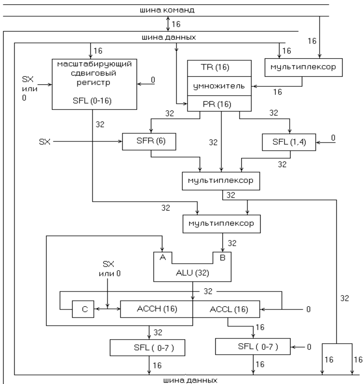
Рисунок 10 - Центральное арифметико-логическое устройство (CALU)
