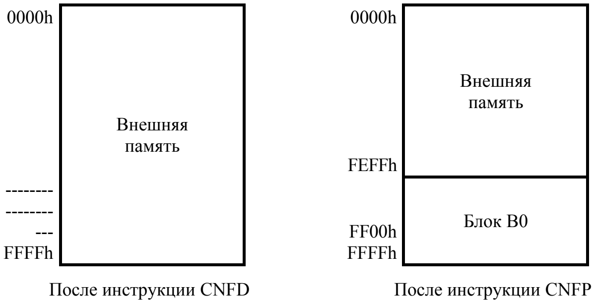
Рисунок 4 - Карты программной памяти ИС 1867BM7Т
