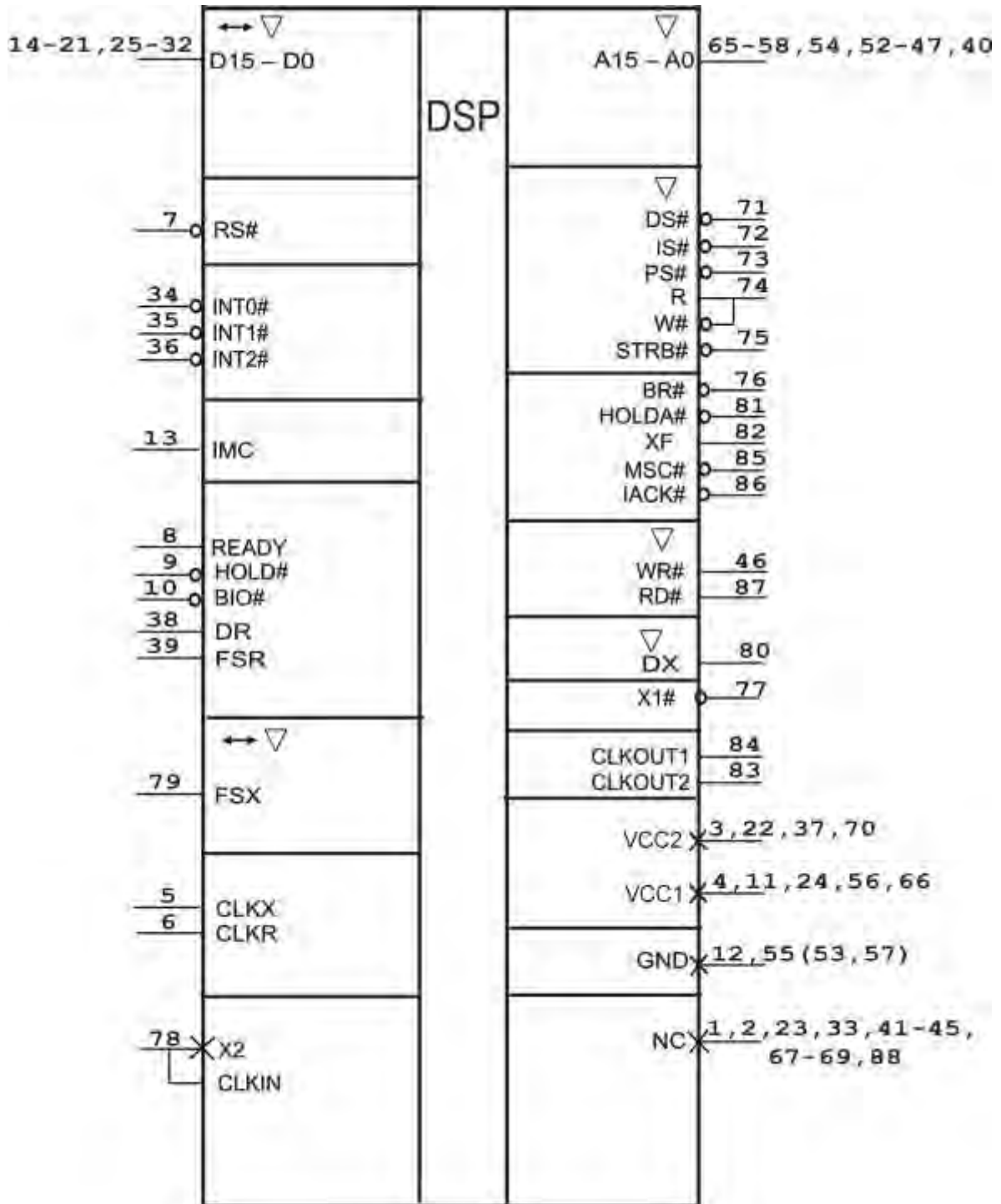
Рисунок 2 – УГО ИС 1867ВМ7Т в корпусе 4235.88-1
