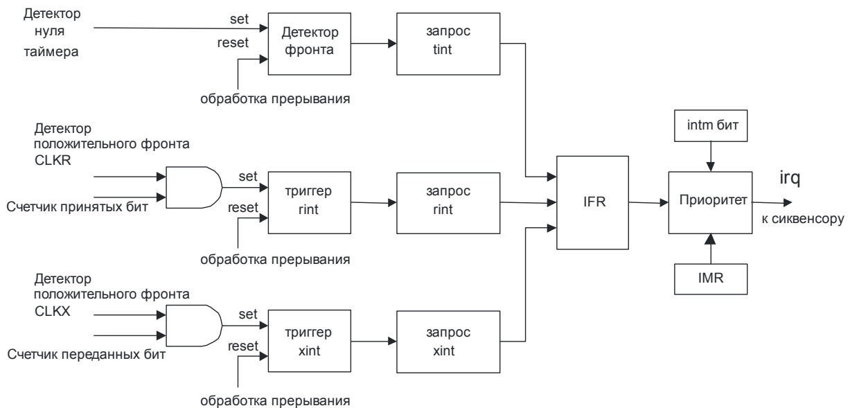
Рисунок 34 - Внутренние прерывания
