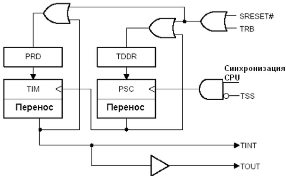
Рисунок 27 - Структурная схема таймера
