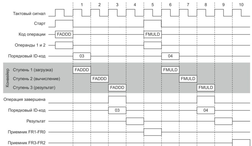
Рисунок 8.3 – Операции сложения и умножения
