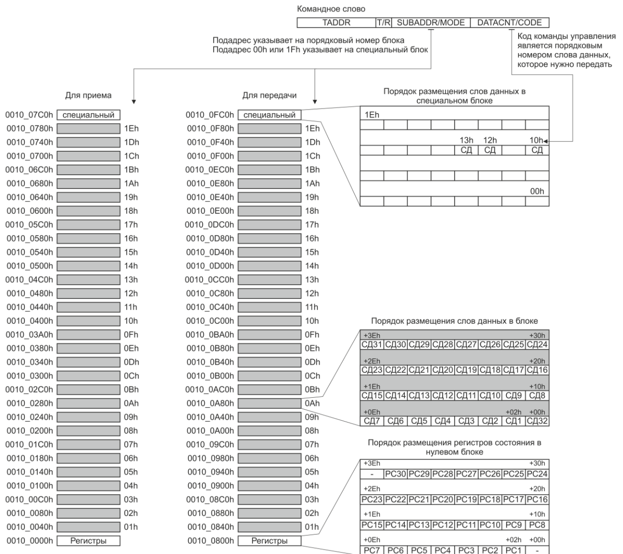
Рисунок 19.3 – Структура памяти сообщений МППО
