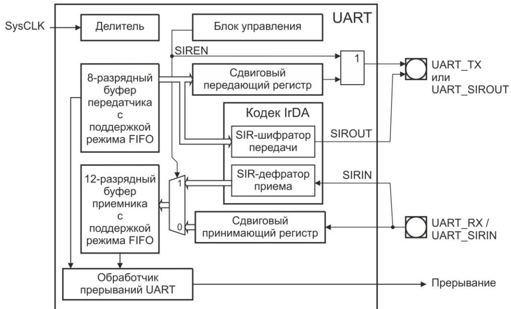
Рисунок 14.1 – Функциональная схема приемопередатчика
