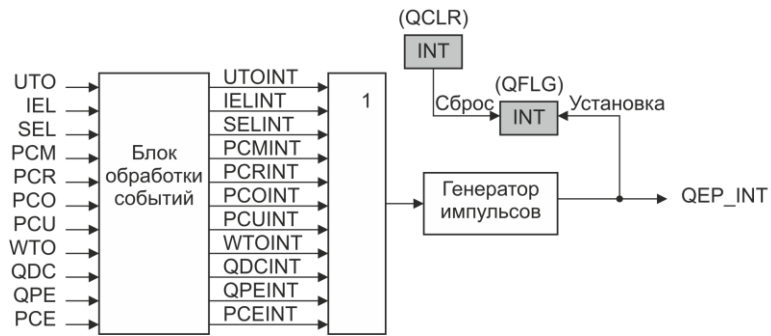
Рисунок 11.12 – Схема системы прерываний
