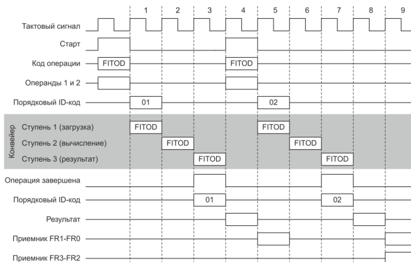
Рисунок 8.2 – Операции преобразования
