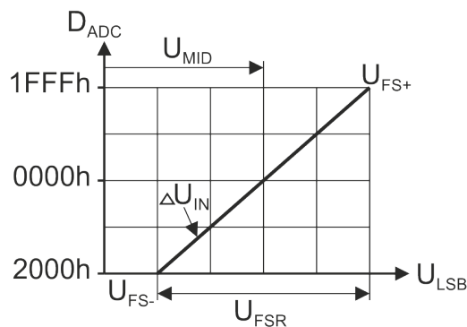
Рисунок 21.2 – Передаточная характеристика АЦП для режима однополярного включения входов (в общем виде)
