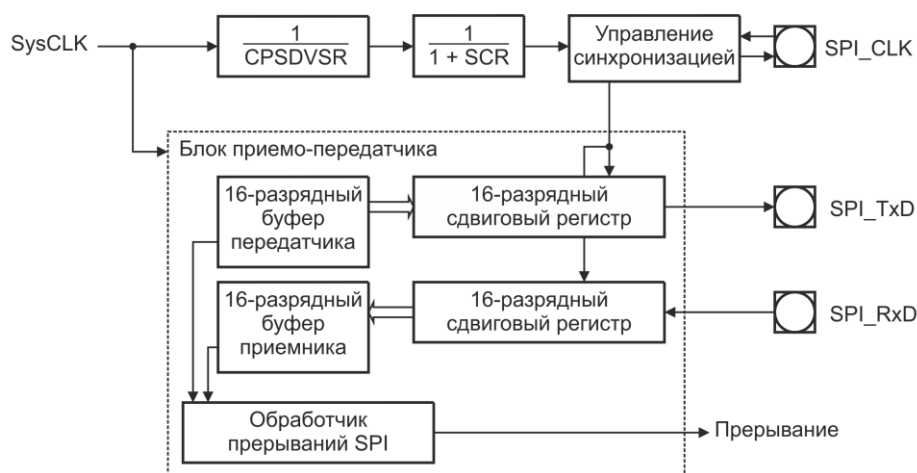
Рисунок 16.1 – Упрощенная функциональная схема контроллера SPI
