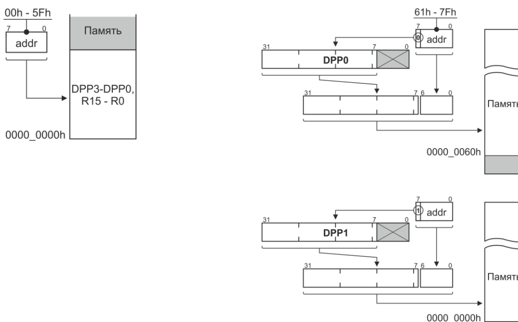
Рисунок 6.1 – Формирование адреса в 16-разрядном режиме
