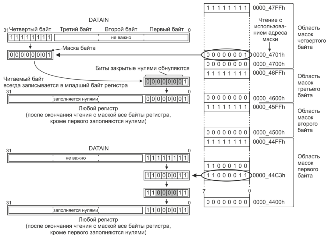
Рисунок 10.6 – Механизм чтения байтов принятых данных порта А с маскированием (на примере младшего и старшего байтов)
