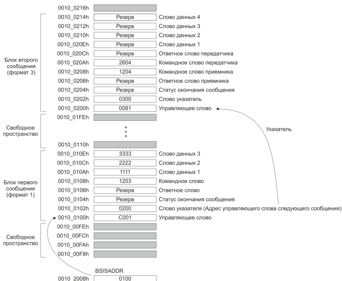
Рисунок 19.2 – Пример размещения двух блоков данных в ОЗУ
