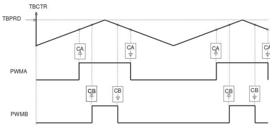
Рисунок 12.10 – Симметричный режим работы при счете вверх-вниз (центрированная модуляция)
