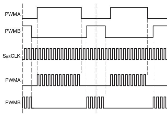
Рисунок 12.15 – Временные диаграммы работы модулятора
