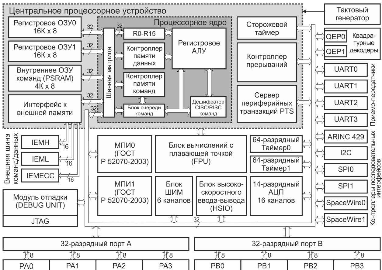
Рисунок 2.1 – Структурная схема микроконтроллера
