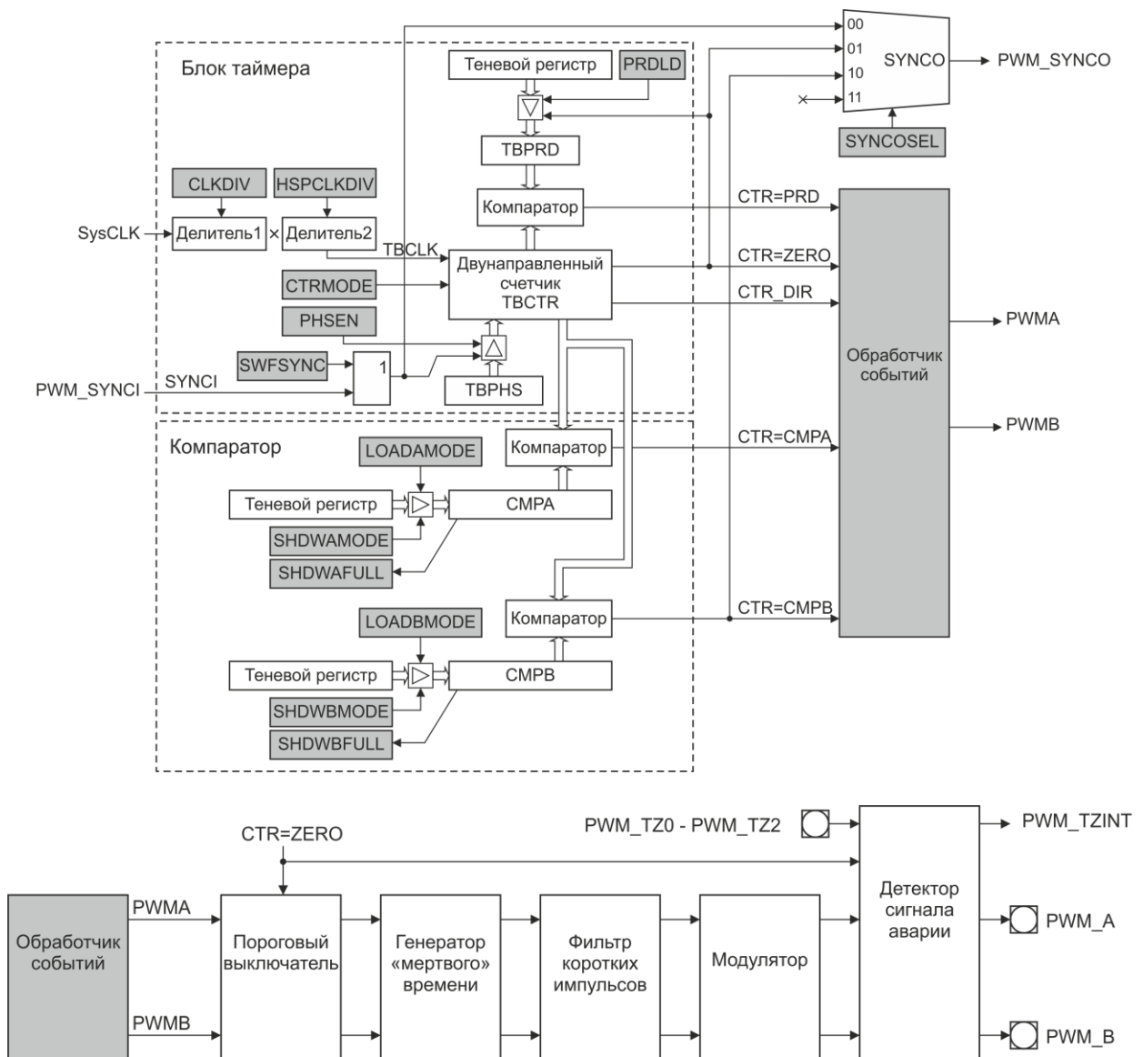
Рисунок 12.1 – Блок ШИМ
