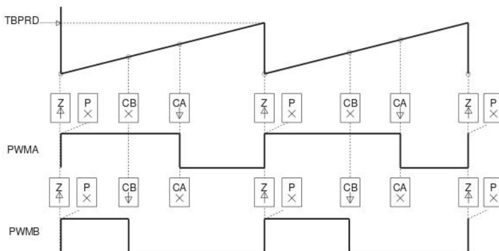
Рисунок 12.9 – Независимый режим работы выходов (фронтальная модуляция)
