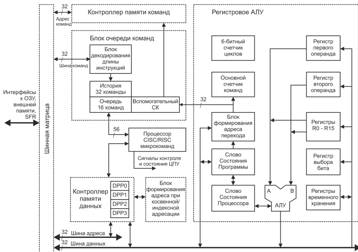
Рисунок 3.1 – Структурная схема ядра микроконтроллера
