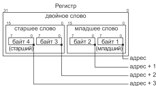
Рисунок 4.1 – Структура регистра
