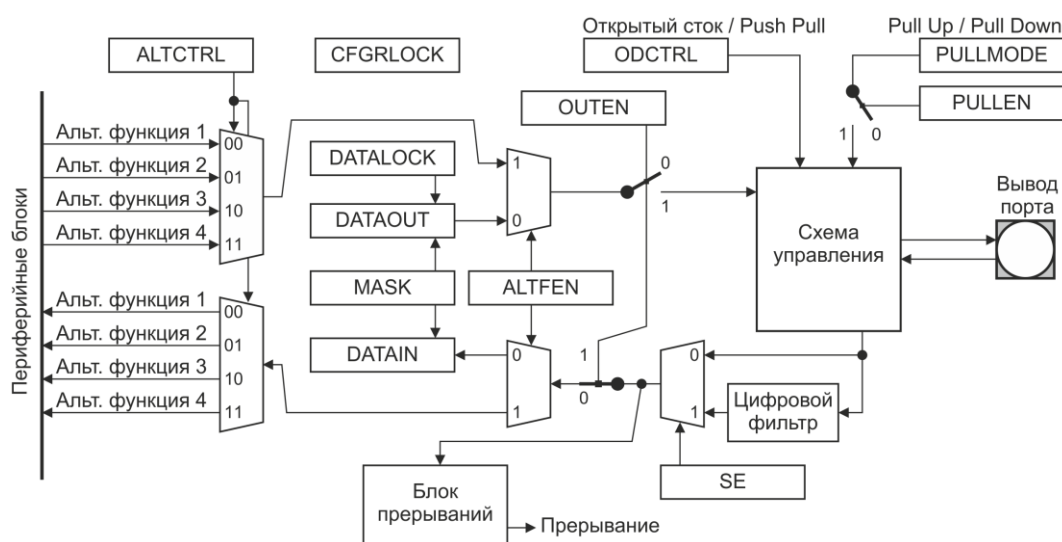
Рисунок 10.1 – Структурная схема вывода порта микроконтроллера и управляющие регистры
