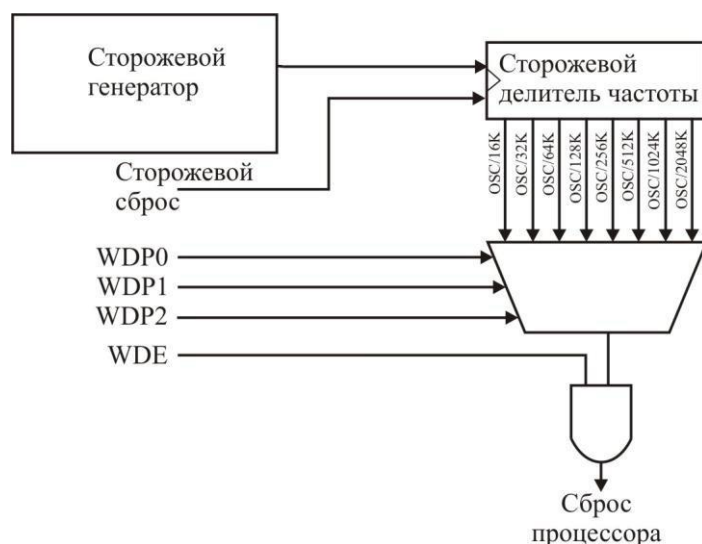
Рисунок 3.19 – Сторожевой таймер
