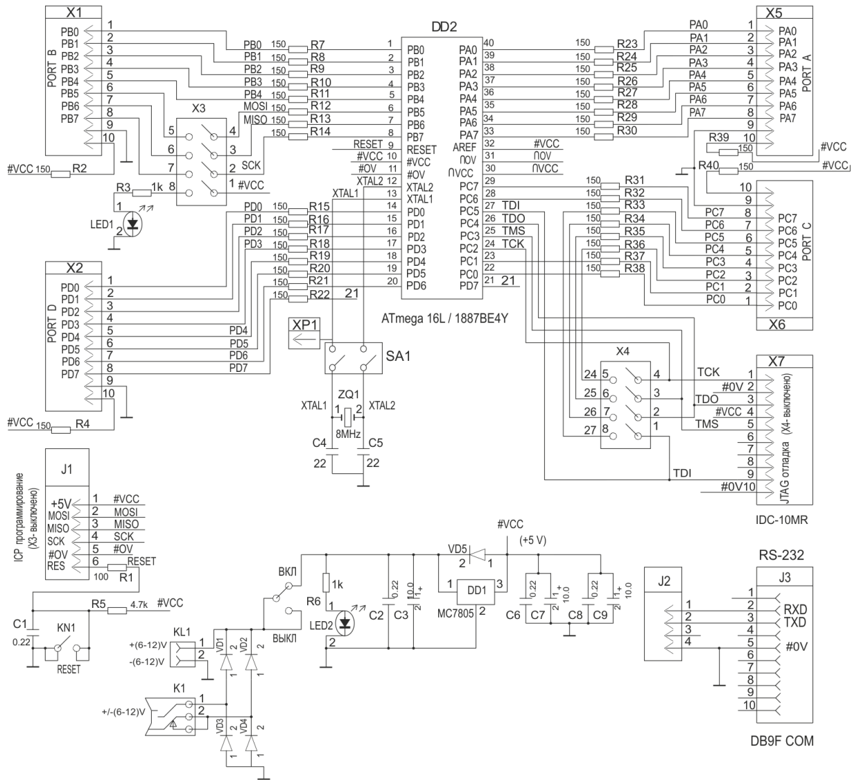
Рисунок В.1 – Схема электрическая основной платы с 40-выводной DIP-колонкой с нулевым усилением для установки микроконтроллеров 1887BE4Y / ATmega16 и макетным полем
