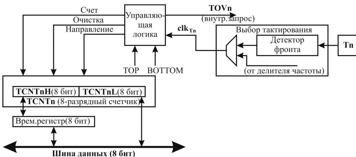
Рисунок 3.39 – Блок-схема модуля счетчика
