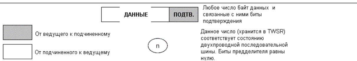
Рисунок 3.91 – Форматы и состояния в режиме подчиненного передатчика
