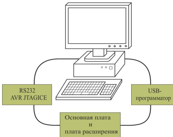
Рисунок 6.1 – Блок-схема устройства
