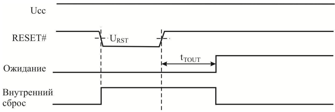
Рисунок 3.16 – Внешний сброс во время работы
