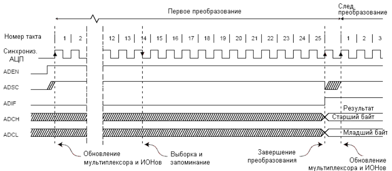
Рисунок 3.99 – Временная диаграмма работы АЦП при первом преобразовании в режиме одиночного преобразования
