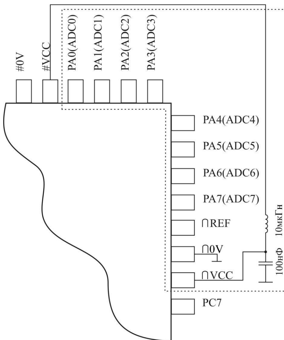
Рисунок 3.103 – Подключение питания АЦП
