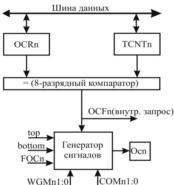
Рисунок 3.53 – Блок-схема модуля сравнения выхода
