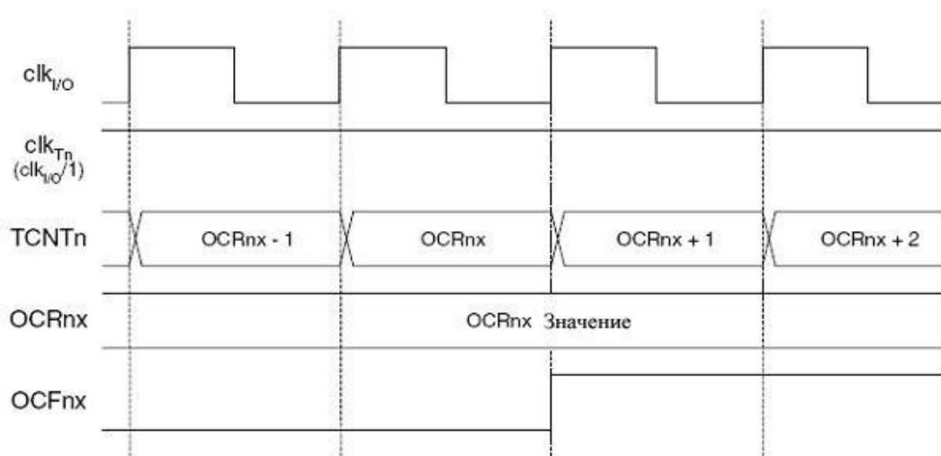
Рисунок 3.47 – Временная диаграмма таймера/счетчика, установка OCF1x без предварительного деления частоты
