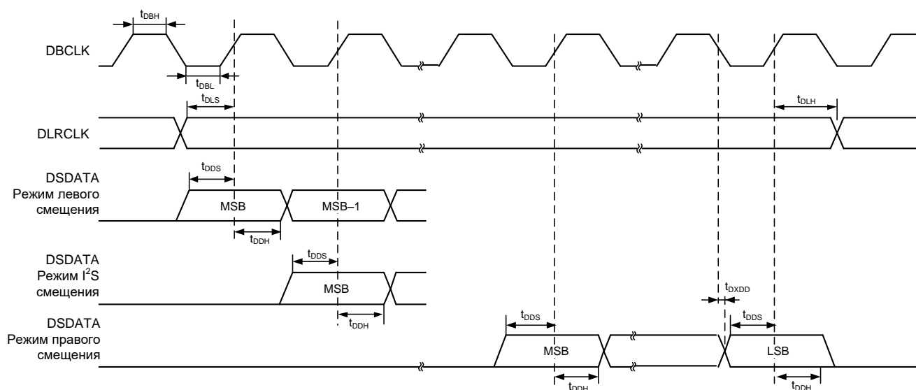
Рисунок 3.10 – Временная диаграмма сигналов последовательного интерфейса данных ЦАП
