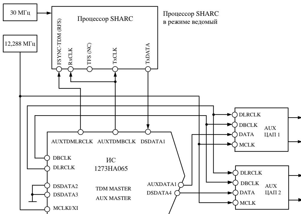
Рисунок 3.9 – Пример соединения микросхемы 1273HA065 с процессором SHARC в режиме AUX (микросхема в режиме TDM-ведущий или AUX-ведущий)
