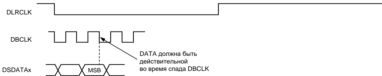
Рисунок 5.2 – Конвейерный режим передачи последовательных данных по I 2 S
