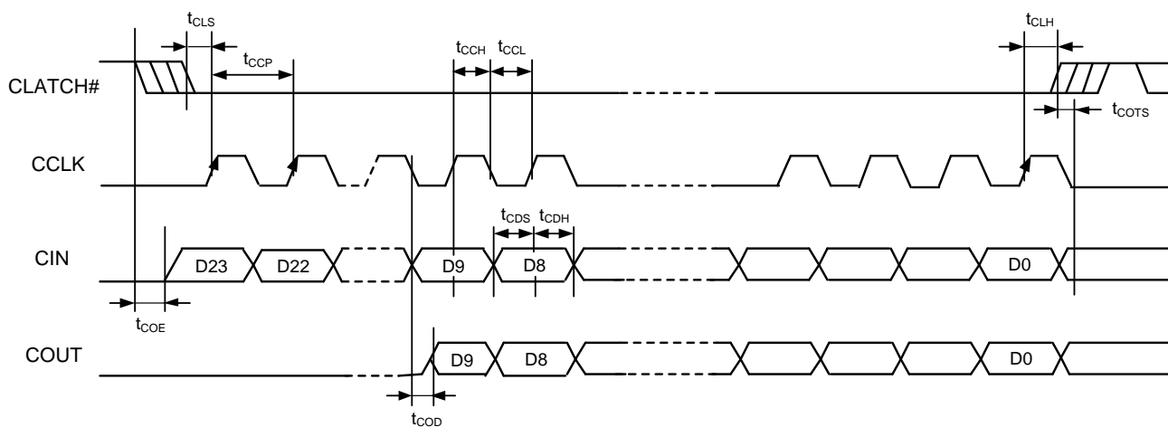
Рисунок 3.2 – Формат сигналов SPI микросхемы 1273HA065
