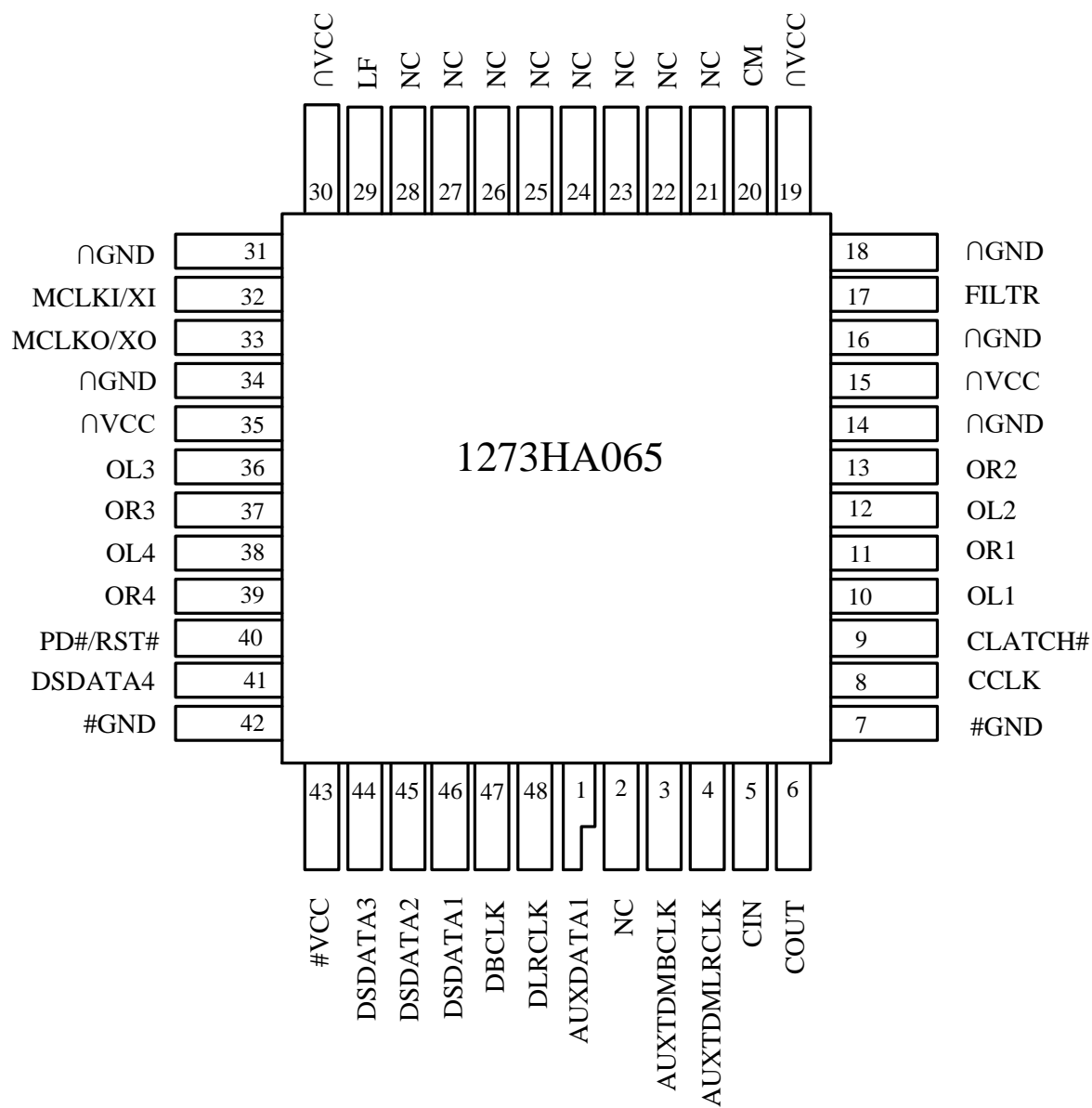
Рисунок 3.12 – Конфигурация выводов микросхемы 1273HA065
