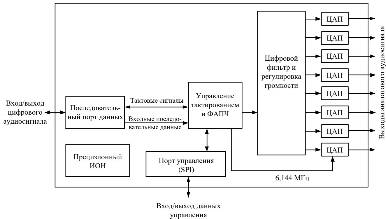
Рисунок 3.1 – Структурная схема микросхемы 1273HA065
