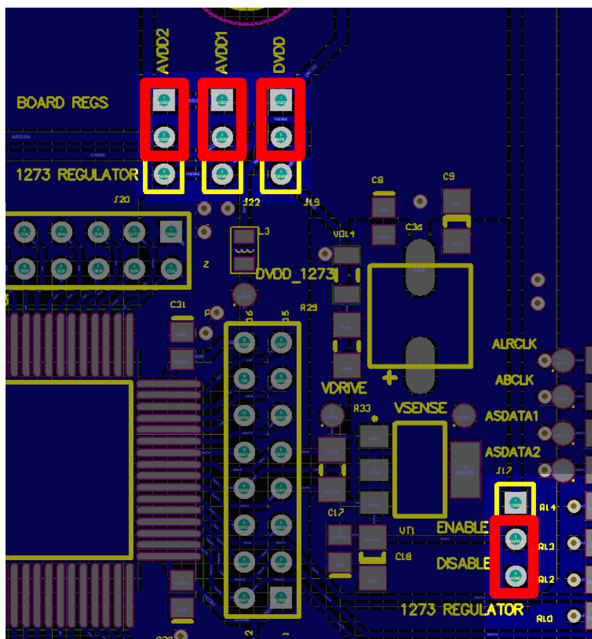
Рисунок 5 – Конфигурация переключиков для работы от стабилизаторов на плате
