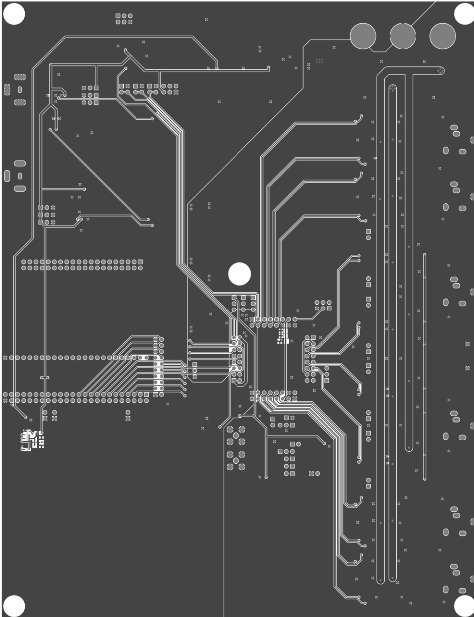
Рисунок 3 – Слой нижней стороны демонстрационной платы (слой металла)
