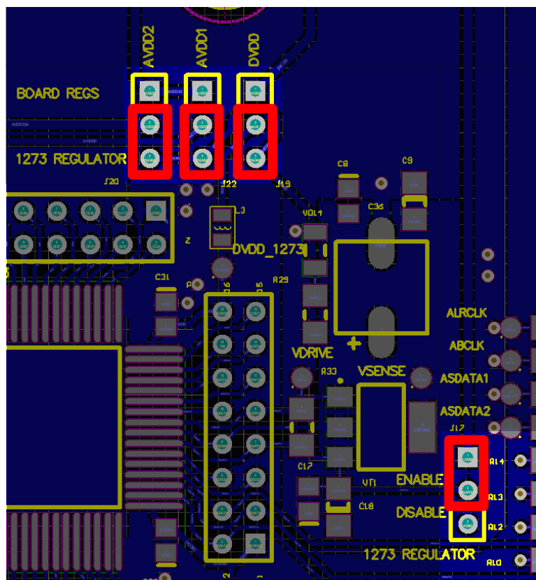
Рисунок 6 – Конфигурация переключек для работы от внутреннего стабилизатора ИС 1273НА054
