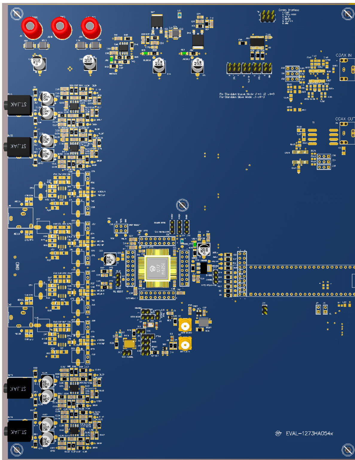
Рисунок 4 – Внешний вид демонстрационной платы
