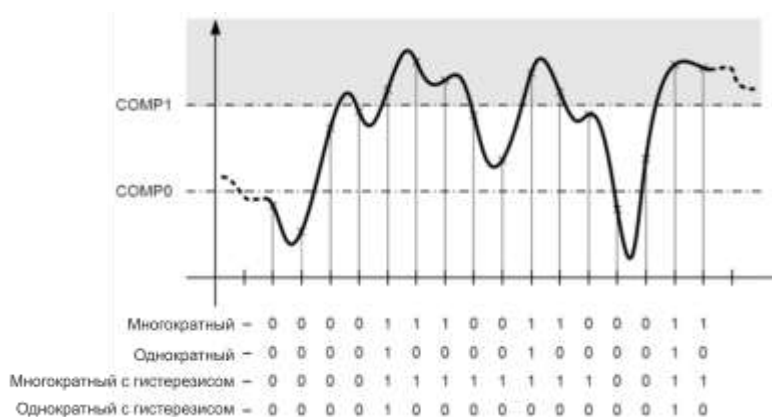
Рисунок 21.11 – Функционирование триггера при СТС = 11h
