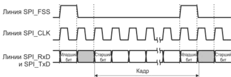
Рисунок 16.8 – Передача кадров данных в интерфейсе SSI
