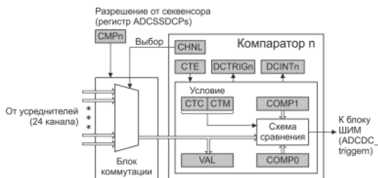
Рисунок 21.8 – Компаратор
