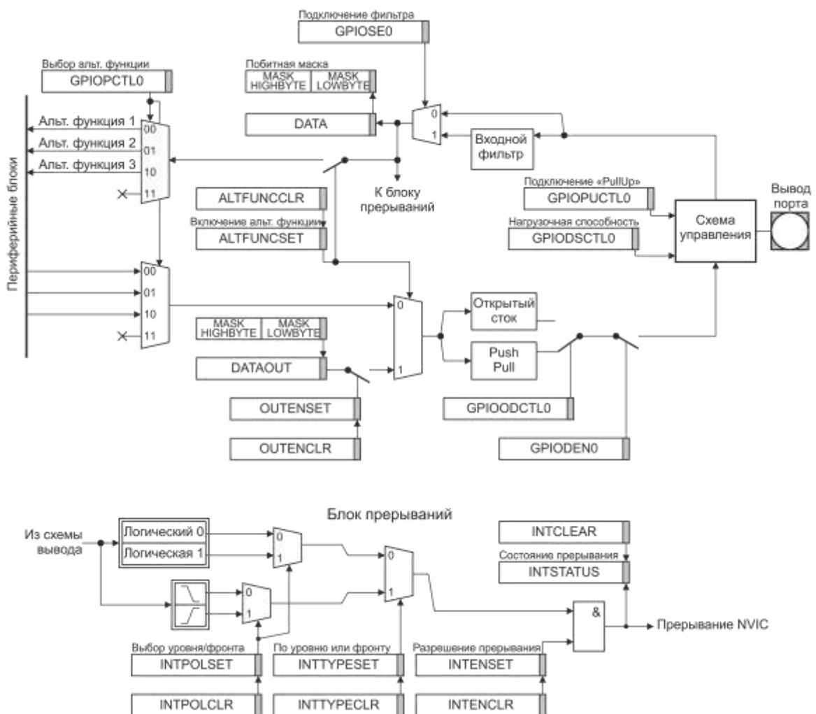
Рисунок 10.1 – Вывод цифрового порта А микроконтроллера и управляющие регистры
