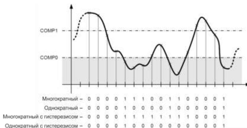
Рисунок 21.9 – Функционирование триггера при СТС = 00h
