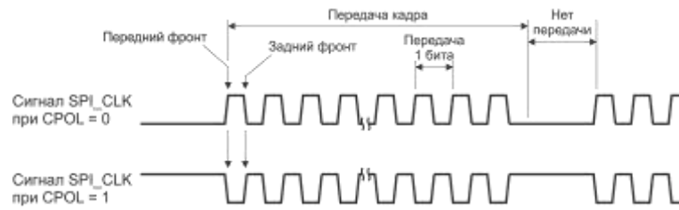
Рисунок 16.2 – Сигнал синхронизации SCK при разных состояниях бита CPOL
