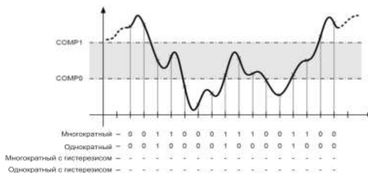
Рисунок 21.10 – Функционирование триггера при СТС = 01h
