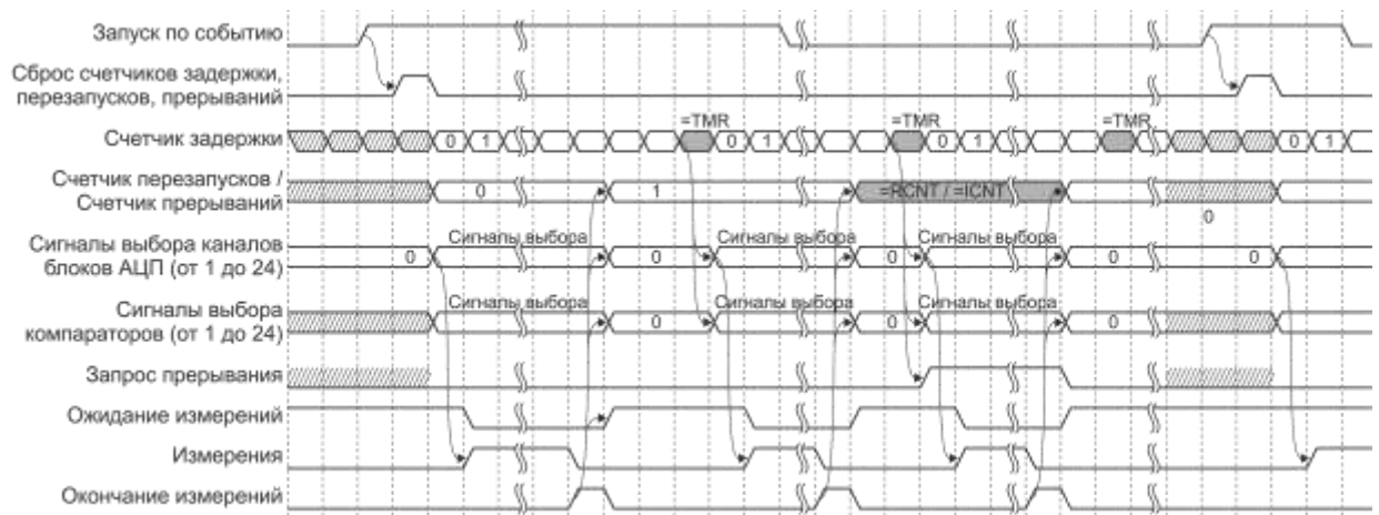
Рисунок 21.3 – Диаграмма работы секвенсора
