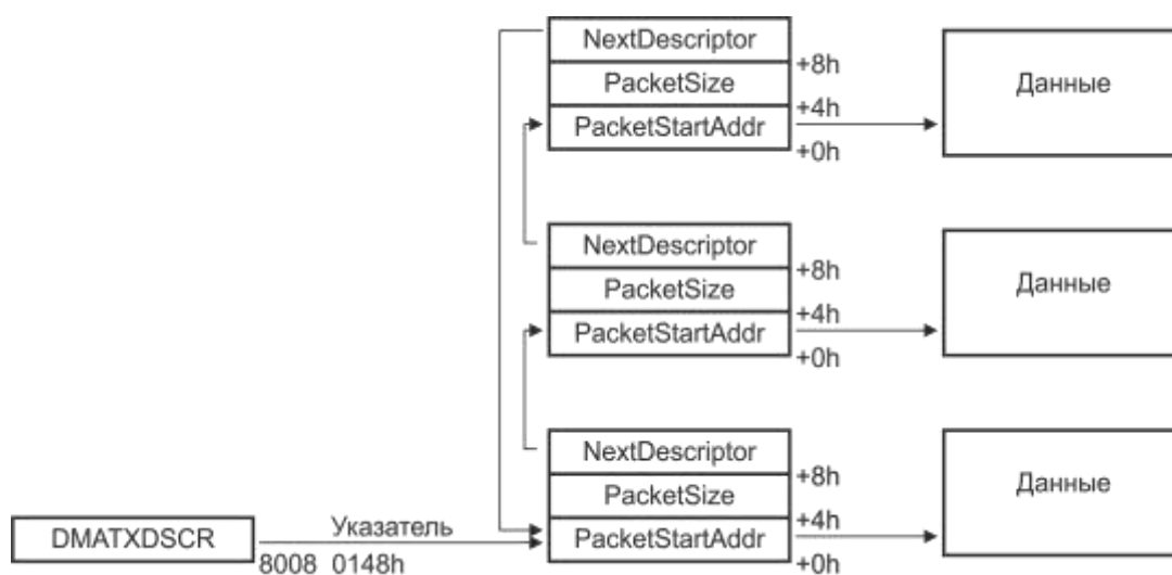
Рисунок 19.1 – Кольцевой буфер с Тх-дескрипторами
