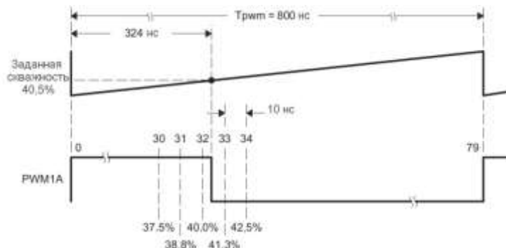
Рисунок 14.21 – Пример работы блока ШИМ высокого разрешения
