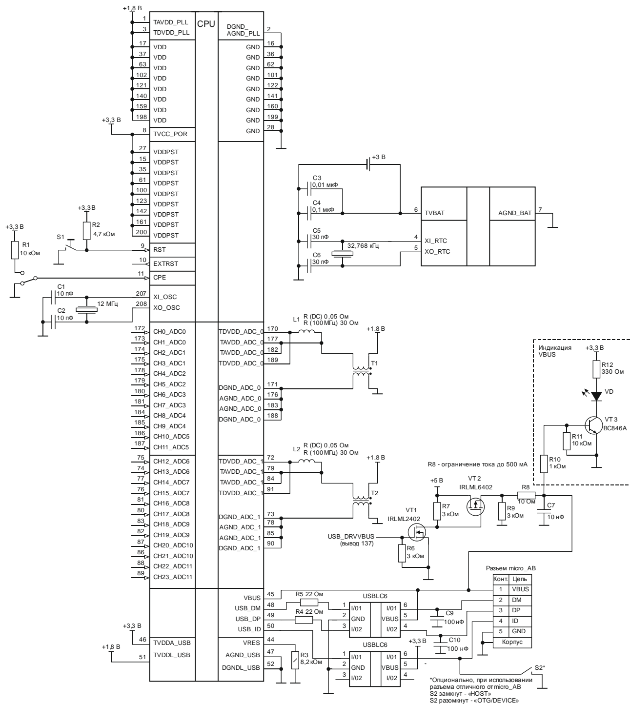
Рисунок Д.1, лист 1 – Пример типовой схемы включения МК K1921BK01T и K1921BK02T
