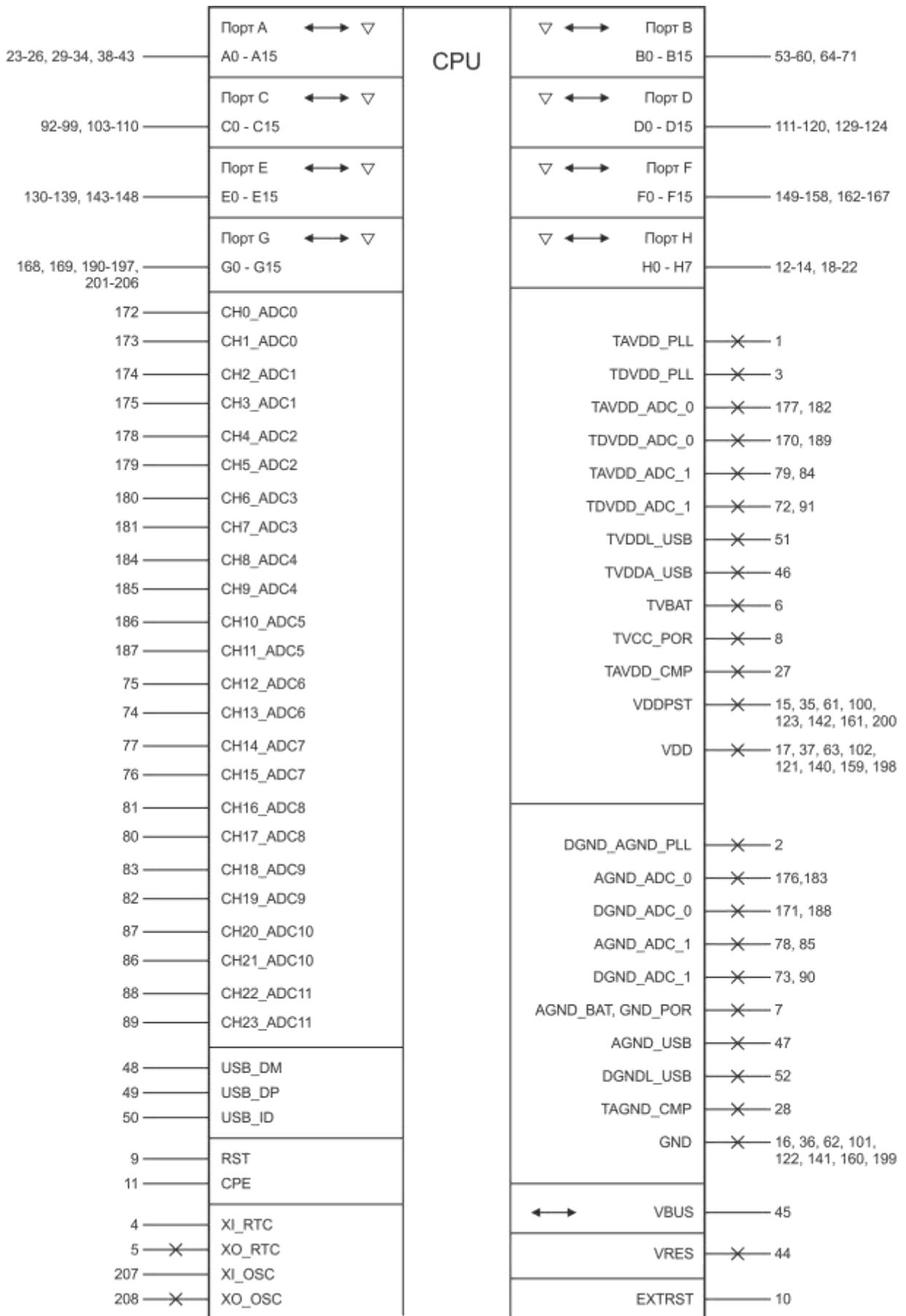
Рисунок 2.2 – Условное графическое изображение микросхем (альтернативные функции выводов портов А, В, С, D, Е, F, G, H указаны в таблице 2.1)
