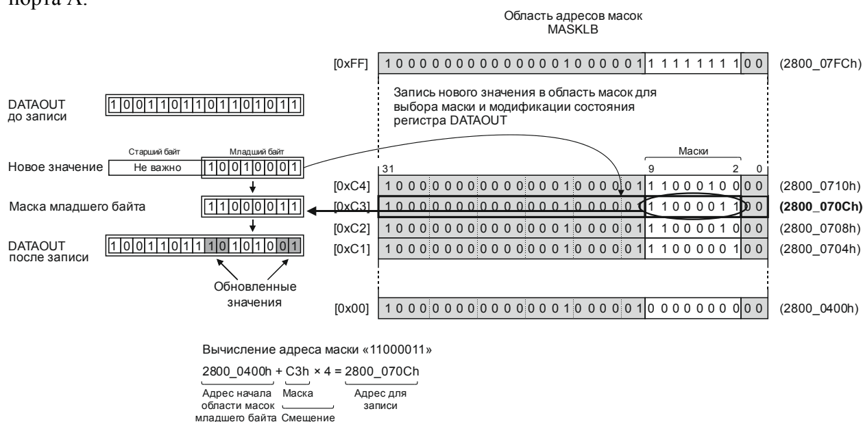
Рисунок 11.4 – Механизм изменения состояния младшего байта порта А с маскированием
