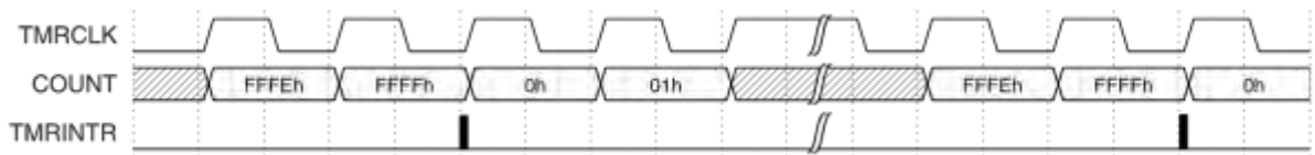
Рисунок 13.5 — Установка флага прерываний в непрерывном режиме
