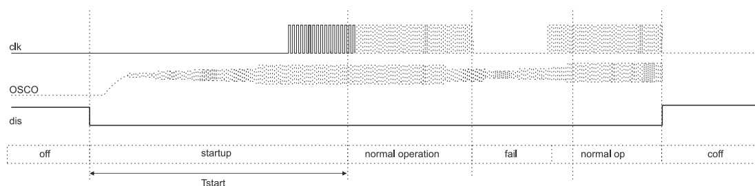
Рисунок 18.2 – Диаграмма старта осциллятора
