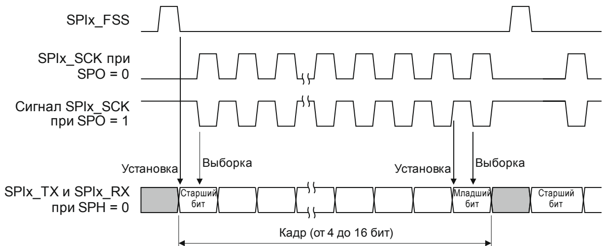
Рисунок 29.5 – Поведение сигналов при непрерывной передаче кадров данных
