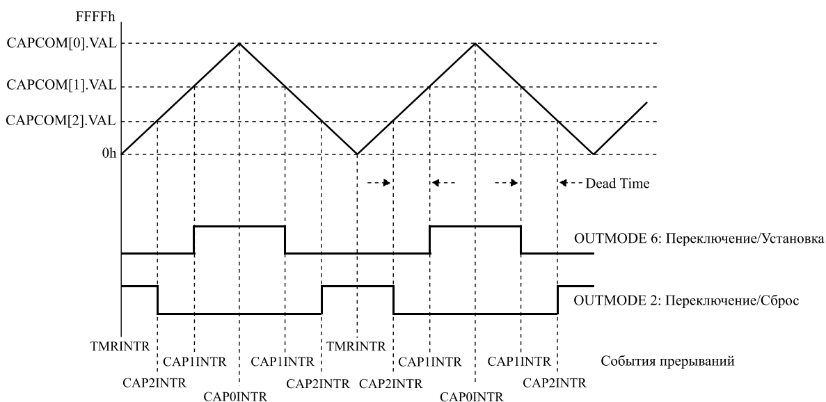
Рисунок 12.9 – Блок вывода в режиме «вверх/вниз»
