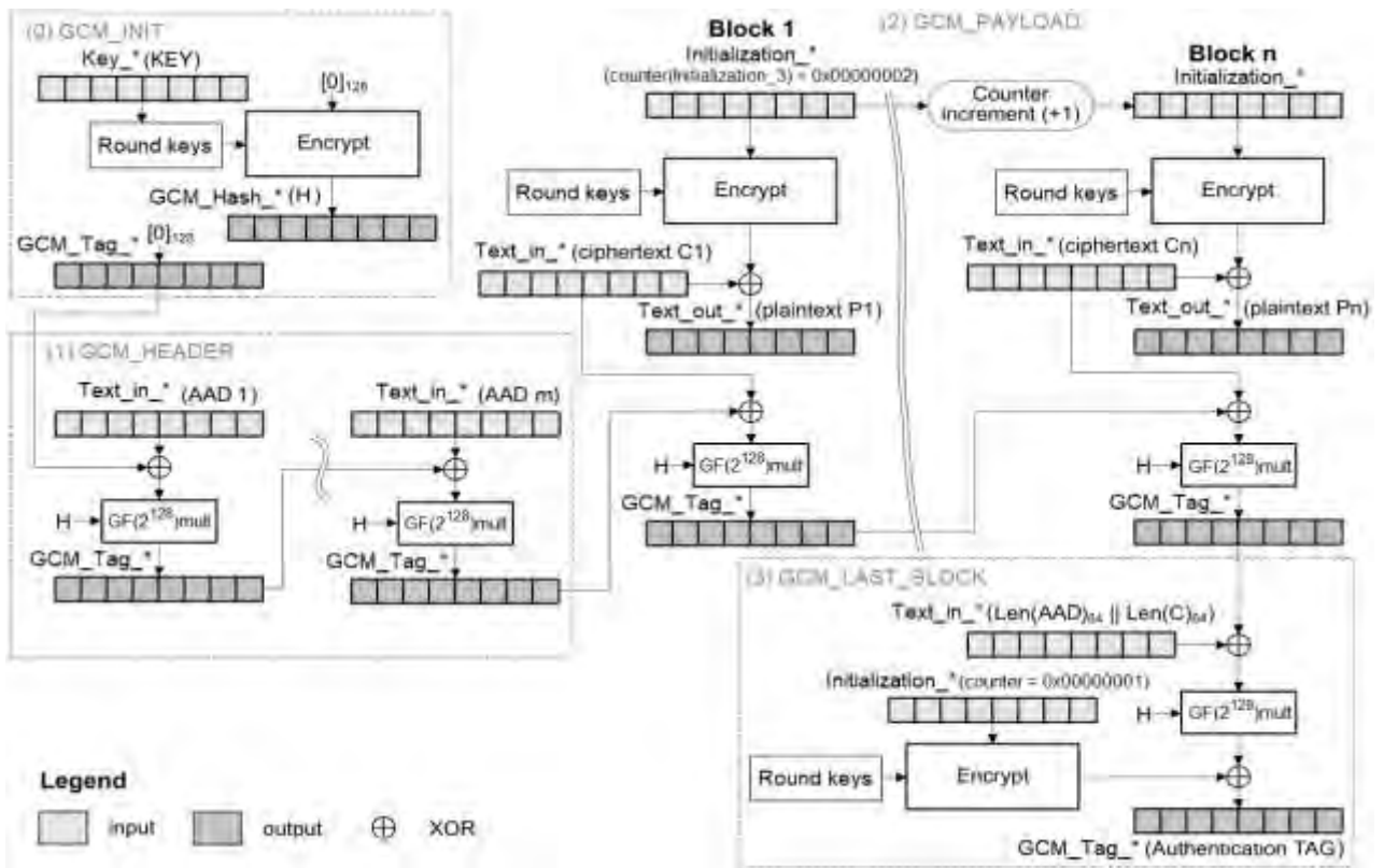
Рисунок 16.12 – Дешифрование сообщения в режиме GCM
