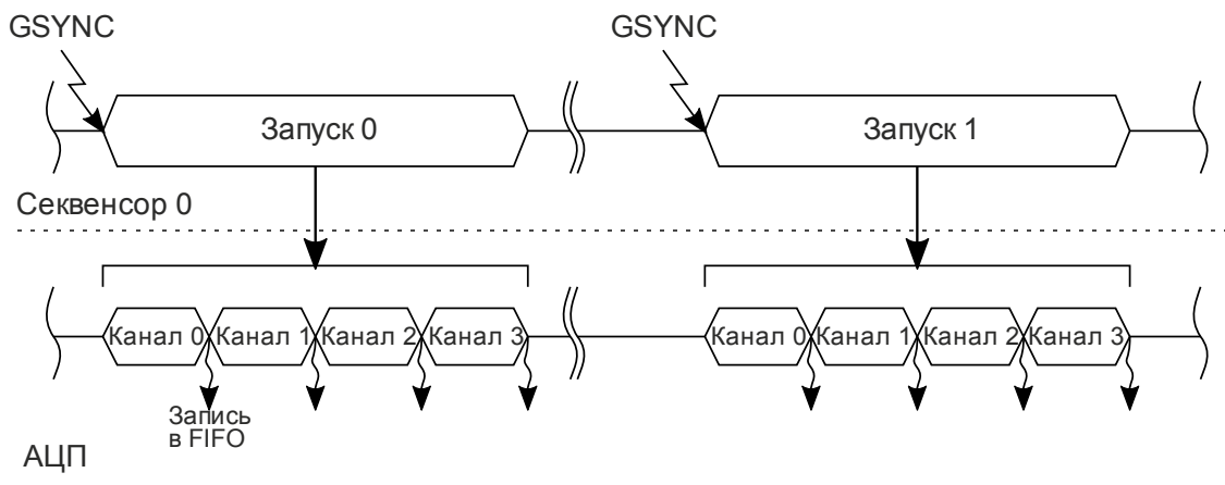
Рисунок 21.19 – Диаграммы программного запуска одного секвенсора
