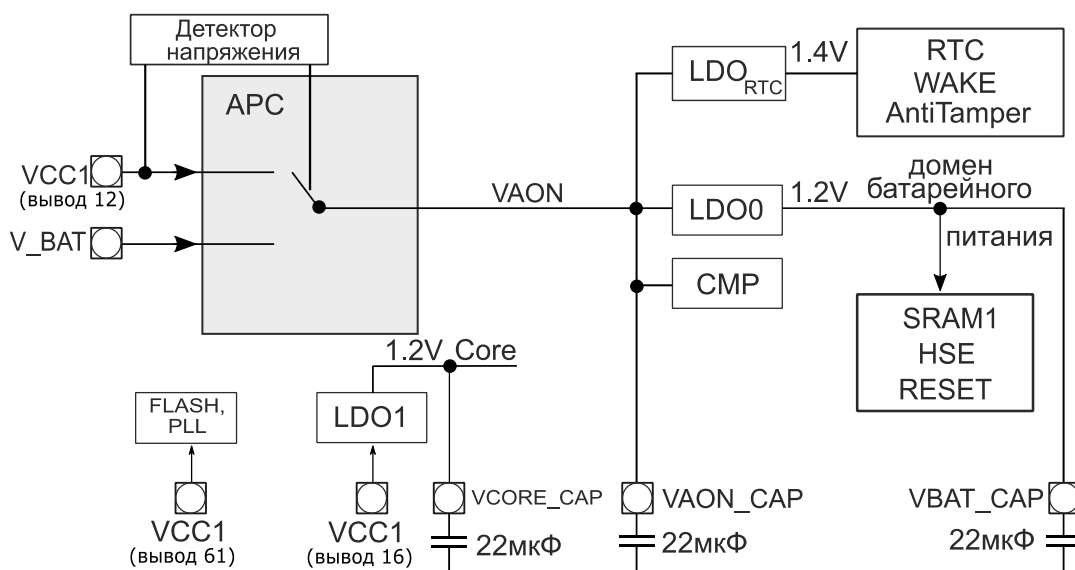
Рисунок 5.1 – Структурная схема питания микроконтроллера
