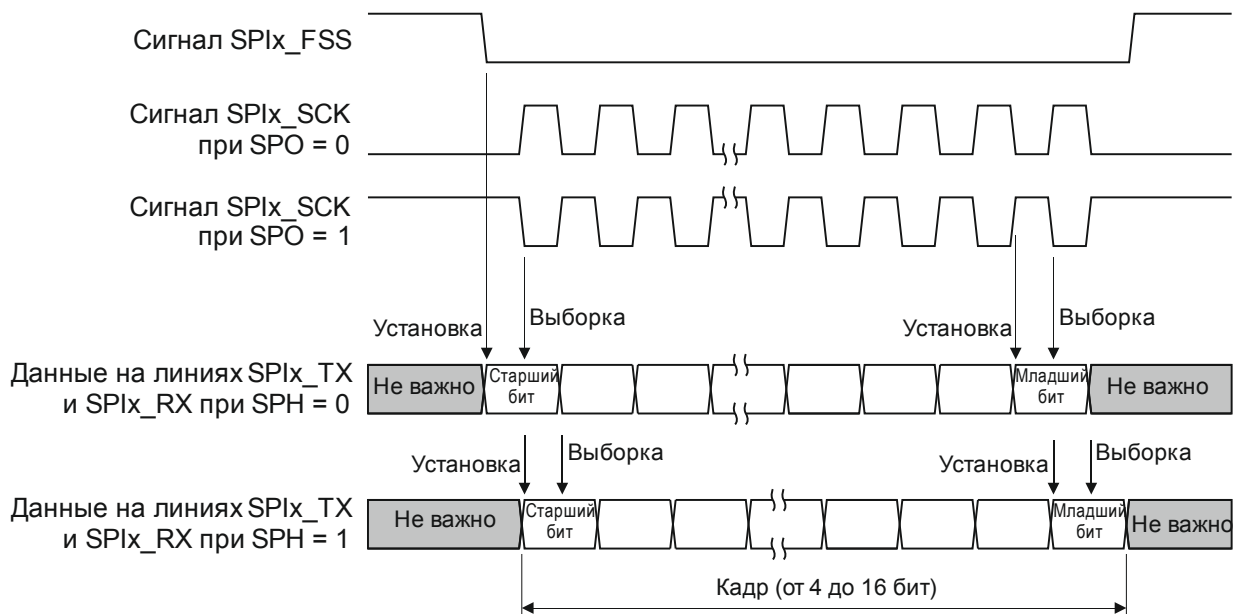
Рисунок 29.4 – Передача кадров данных в интерфейсе SPI
