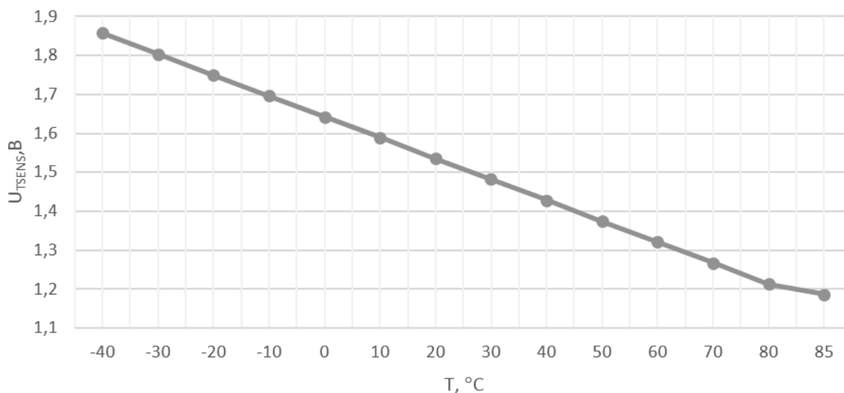
Рисунок 23.2 – График зависимости напряжения на выходе датчика от температуры
