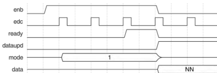
Рисунок 22.2 – Диаграмма переключения внутренних сигналов в режиме 1.
