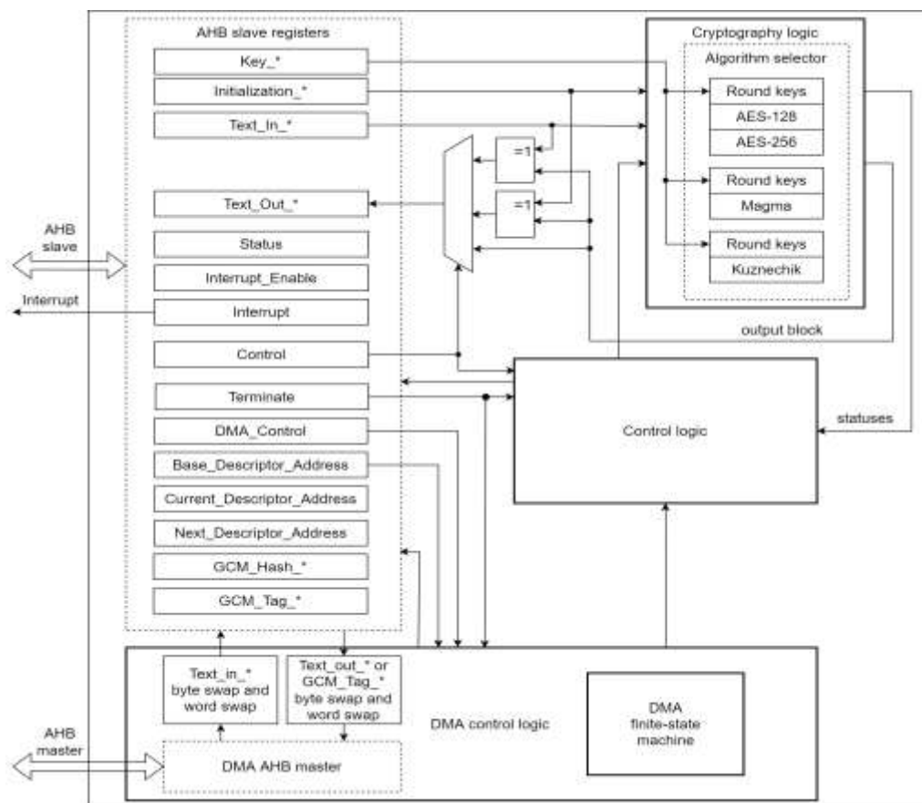
Рисунок 16.1 – Структурная схема блока криптографии
