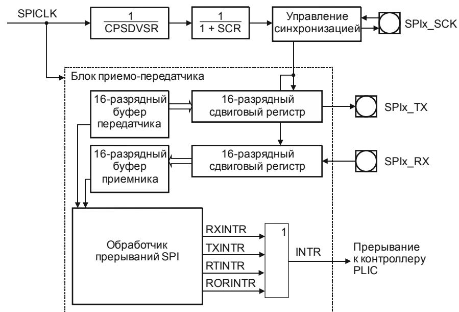
Рисунок 29.1 – Упрощенная функциональная схема контроллера SPI
