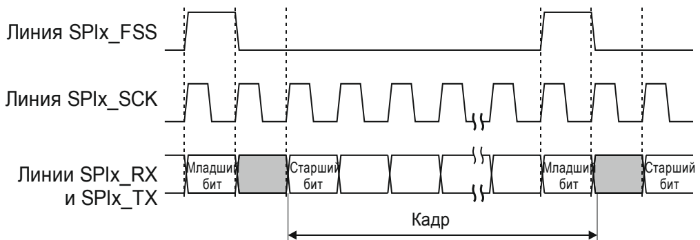
Рисунок 29.9 – Непрерывная передача кадров данных в интерфейсе SSI
