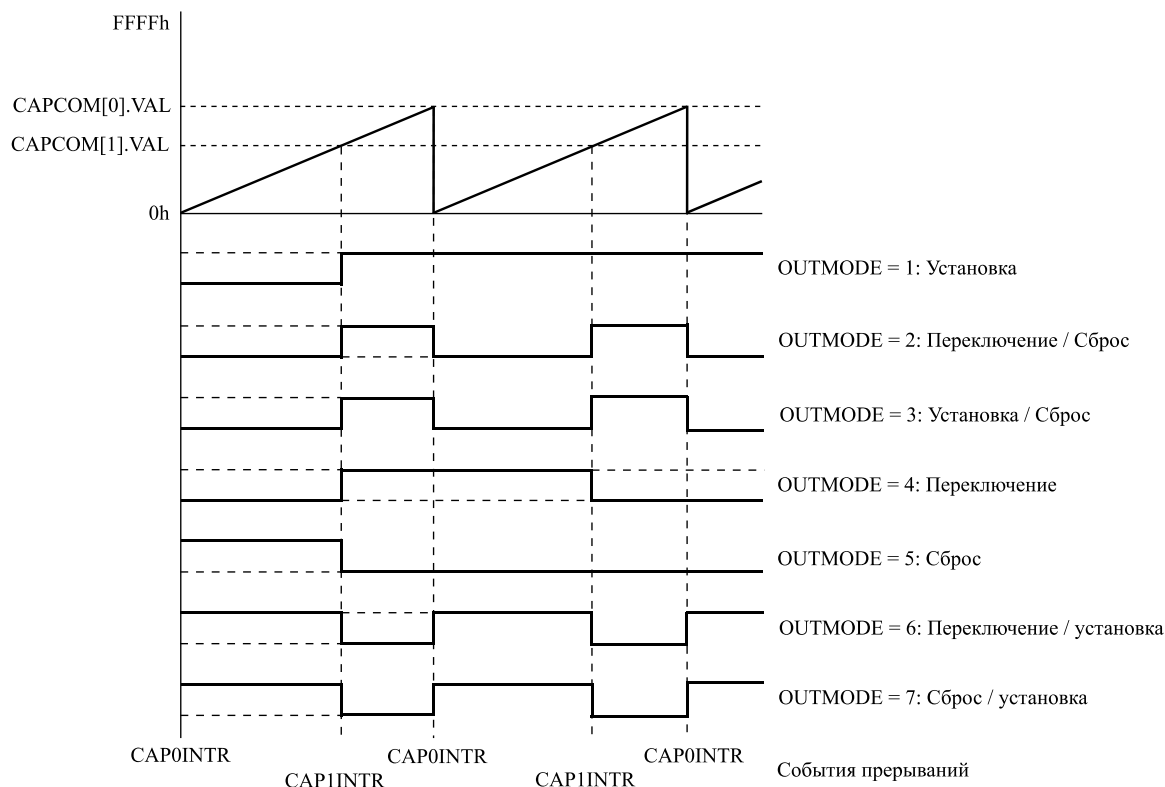
Рисунок 13.12 – пример вывода. Таймер в режиме счета вверх
