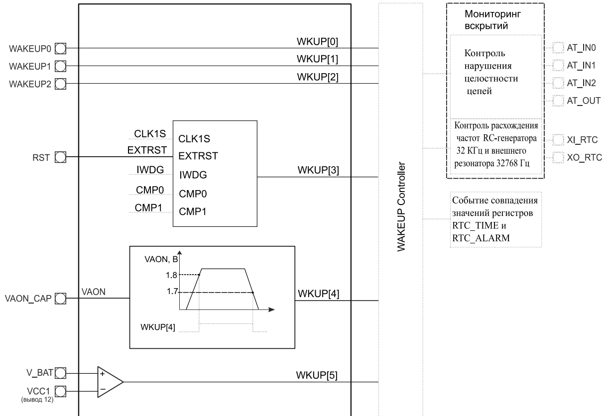
Рисунок 18.3 – Структурная схема контроллера пробуждения WAKE
