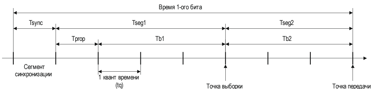
Рисунок 26.14 – Структура одного бита
