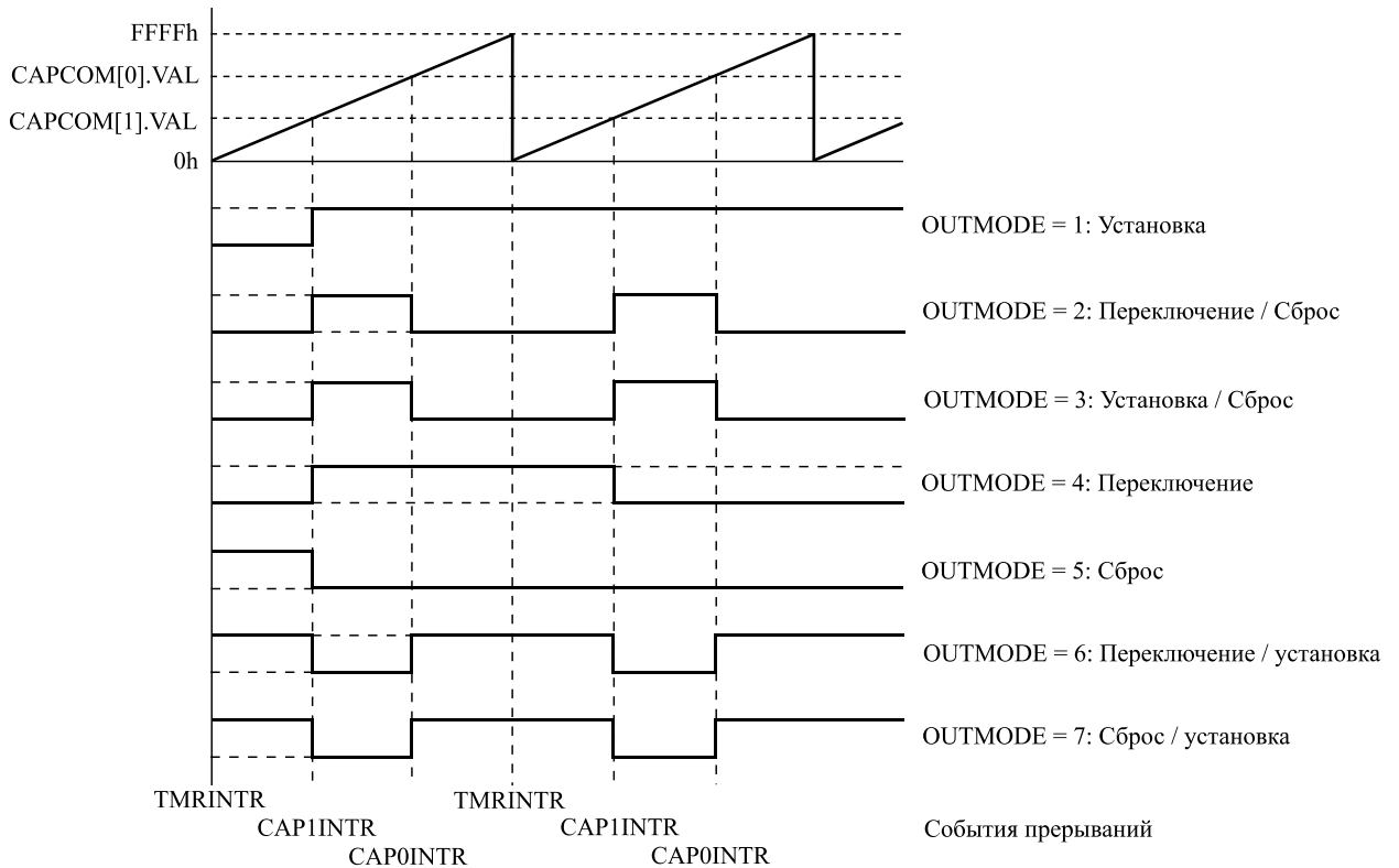
Рисунок 13.13 – пример вывода. Таймер в непрерывном режиме
