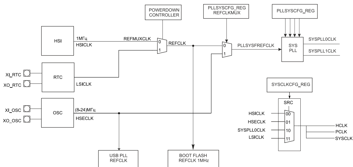
Рисунок 4.1 – Схема синхронизации
