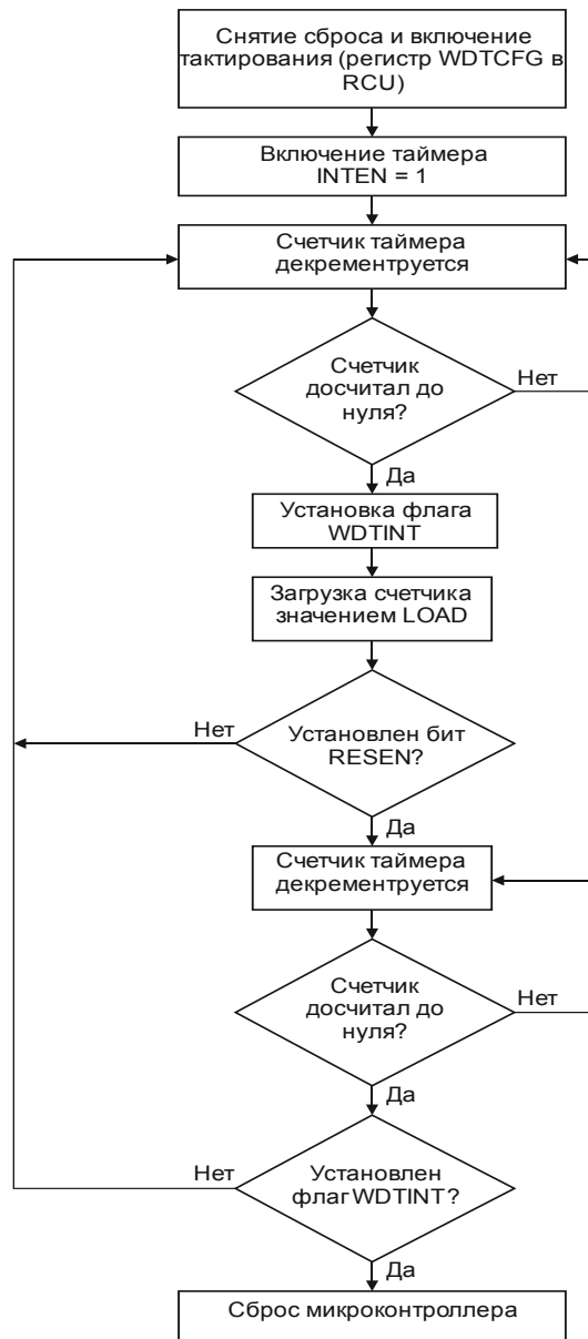
Рисунок 20.1 – Алгоритм работы независимого сторожевого таймера
