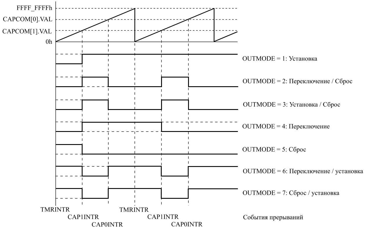
Рисунок 12.13 – пример вывода. Таймер в непрерывном режиме
