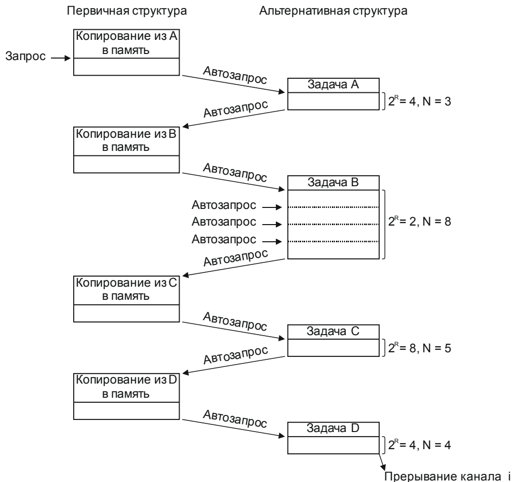
Рисунок 10.4 – Пример функционирования контроллера DMA в режиме «разборка-сборка»
