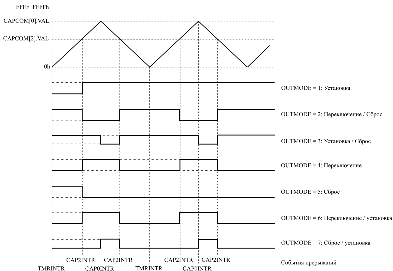
Рисунок 12.14 – пример вывода. Таймер в режиме счета «вверх/вниз»
