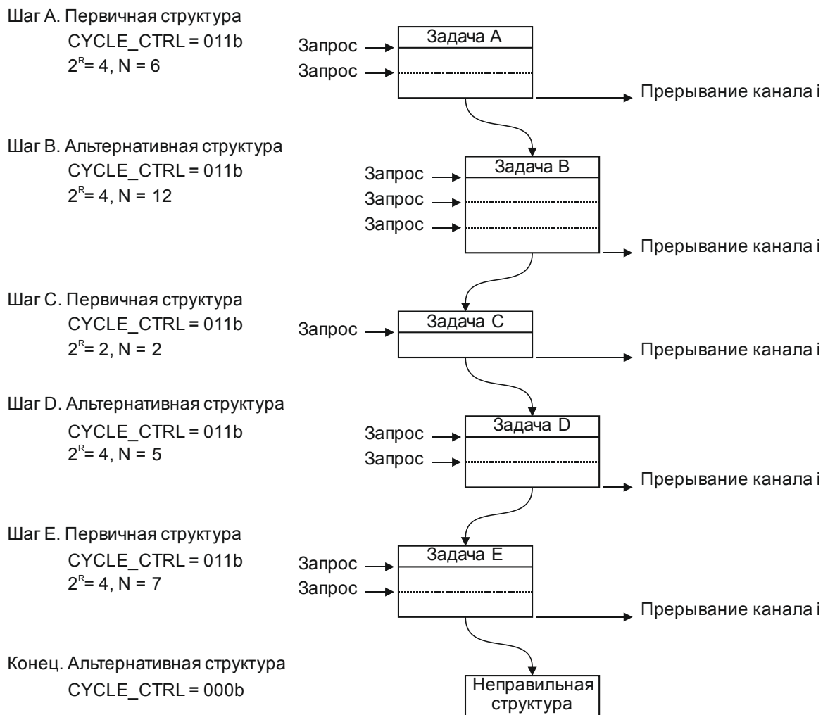
Рисунок 10.3 – Пример функционирования контроллера DMA в режиме «пинг-понг»
