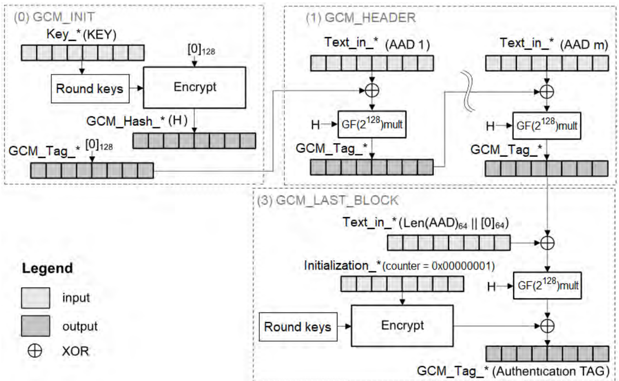
Рисунок 16.13 – Формирование аутентификационного тега в режиме GMAC
