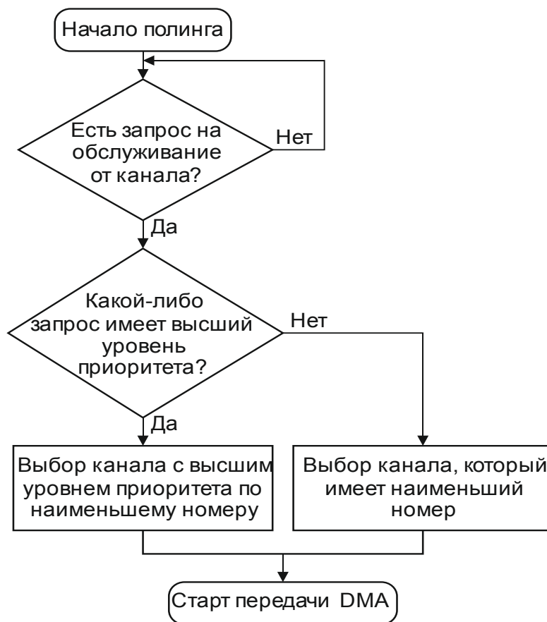
Рисунок 10.2 – Алгоритм выбора (полинга) следующего канала для обслуживания
