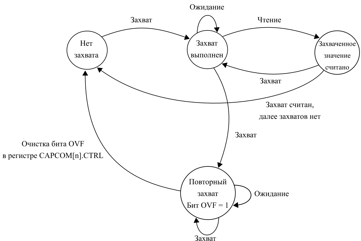
Рисунок 12.11 – Цикл захвата
