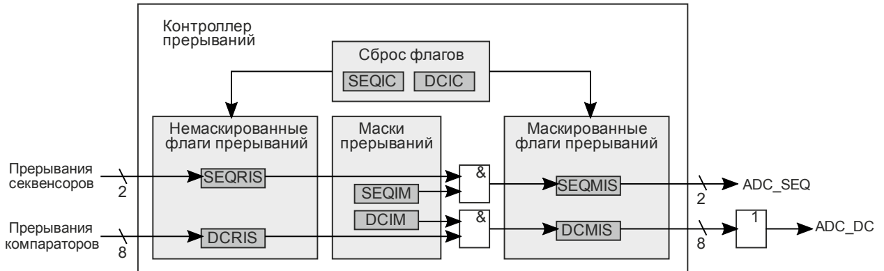
Рисунок 21.18 – Контроллер прерываний
