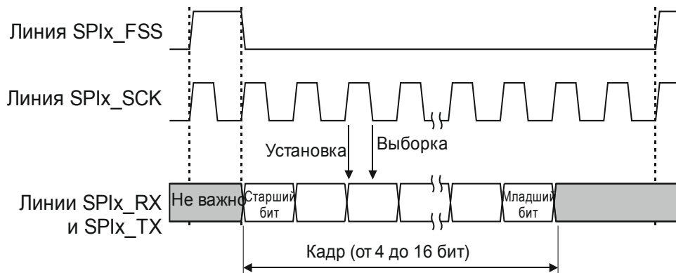
Рисунок 29.8 – Передача кадра данных в интерфейсе SSI
