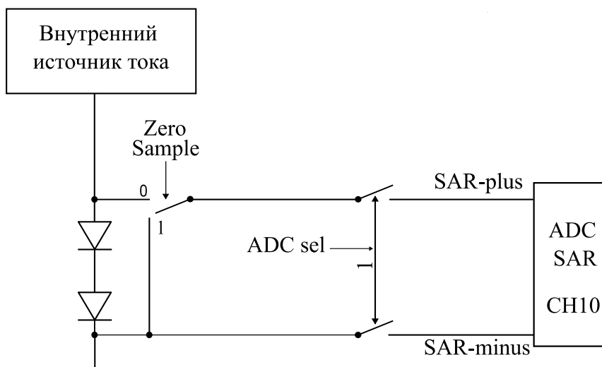
Рисунок 23.1 – Структурная схема датчика температуры
