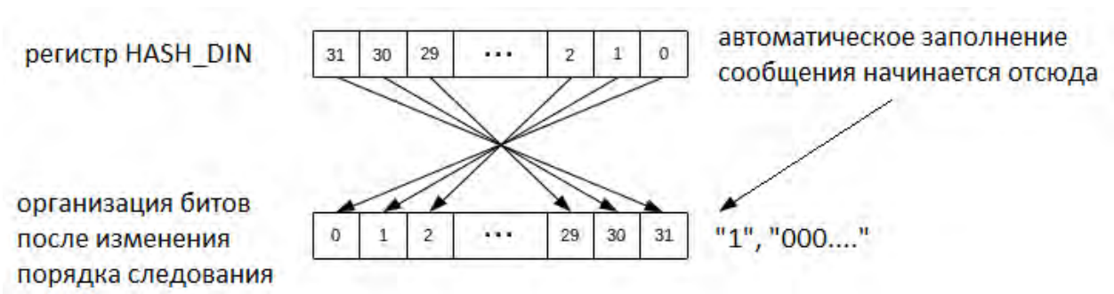
Рисунок 15.2 – Представление входных данных как битовой строки
