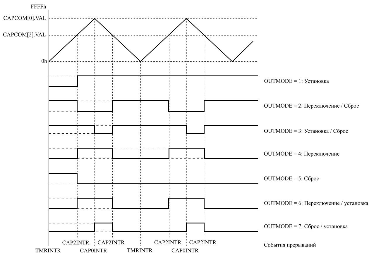
Рисунок 13.14 – пример вывода. Таймер в режиме счета «вверх/вниз»
