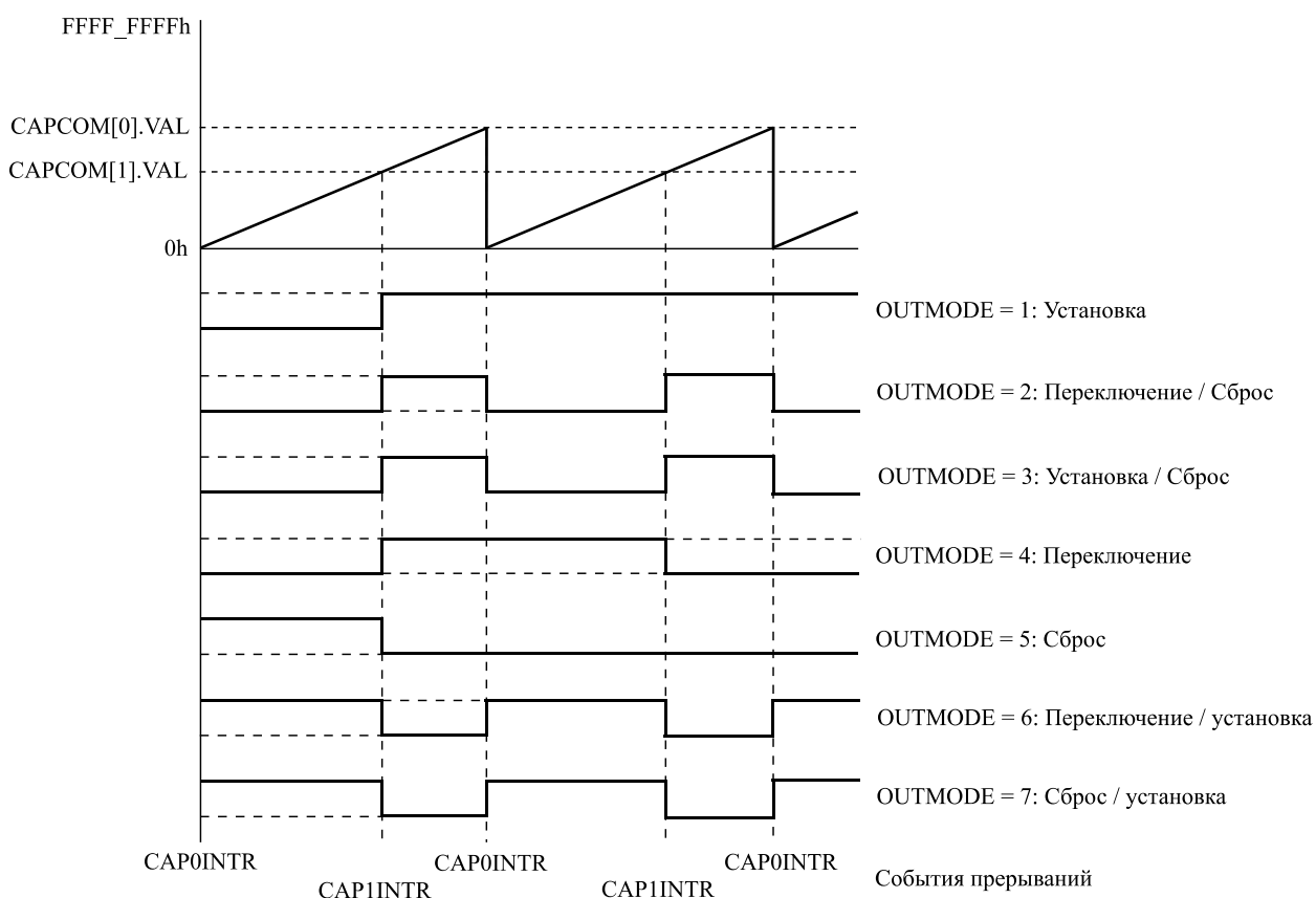
Рисунок 12.12 – пример вывода. Таймер в режиме счета вверх
