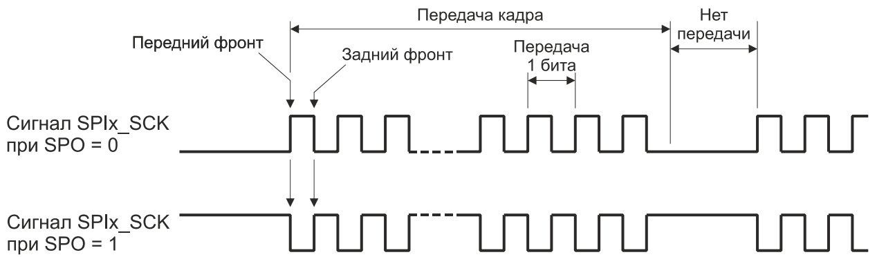
Рисунок 29.3 – Сигнал синхронизации SPIx_SCK при разных состояниях бита SPO
