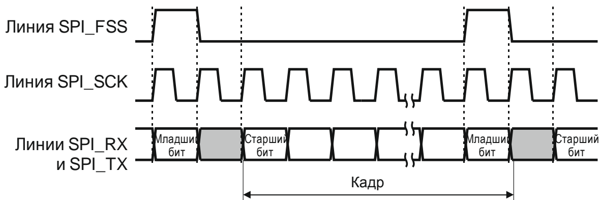
Рисунок 16.8 – Непрерывная передача кадров данных в интерфейсе SSI
