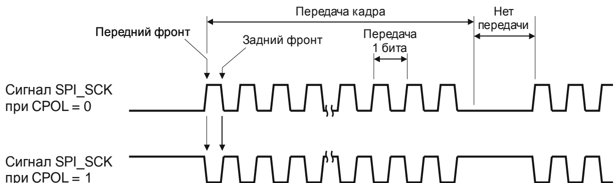
Рисунок 16.2 – Сигнал синхронизации SPI_SCK при разных состояниях бита CPOL. Комбинации битов SPO и SPH задают четыре режима обмена данными, см. рисунок 16.3.
