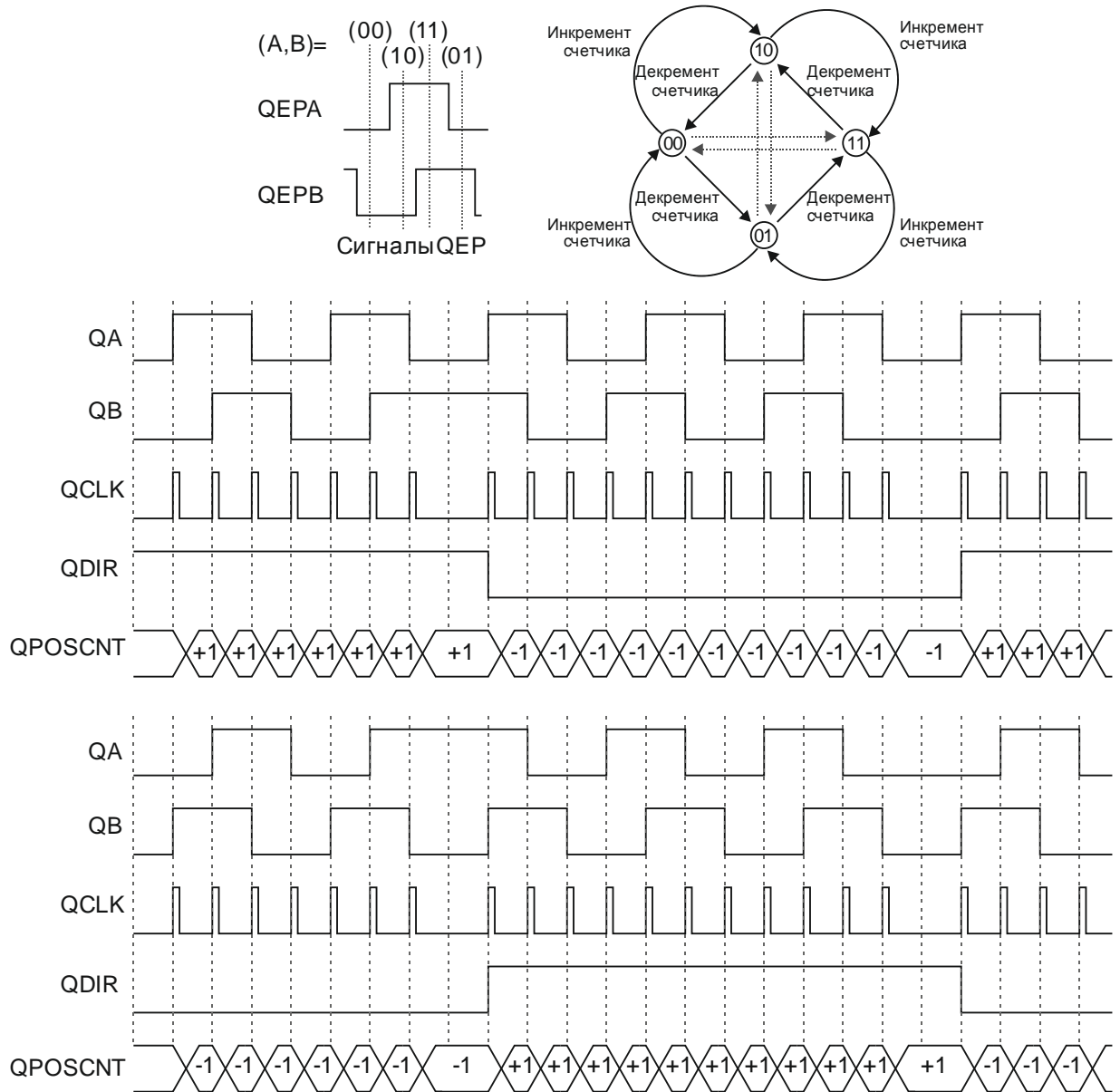
Рисунок 13.4 – Временные диаграммы и автомат состояний работы в квадратурном режиме счета
