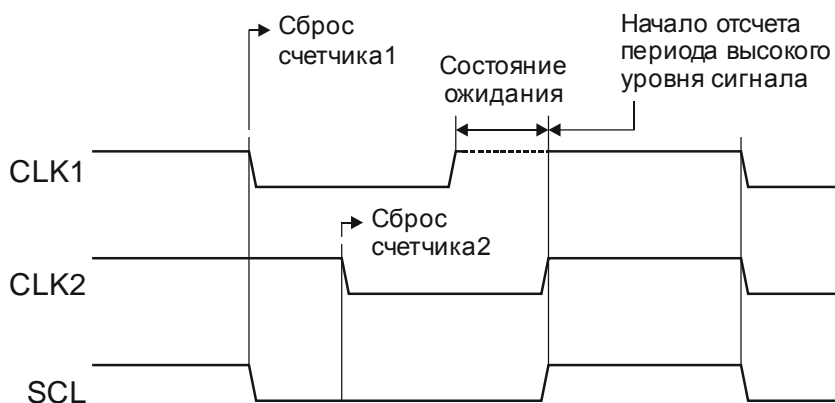
Рисунок 17.5 – Синхронизация
