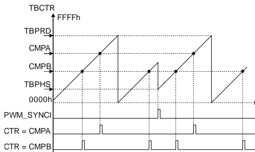
Рисунок 14.6 – Диаграммы работы при счете вверх
