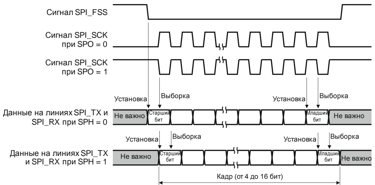
Рисунок 16.3 – Передача кадров данных в интерфейсе SPI
