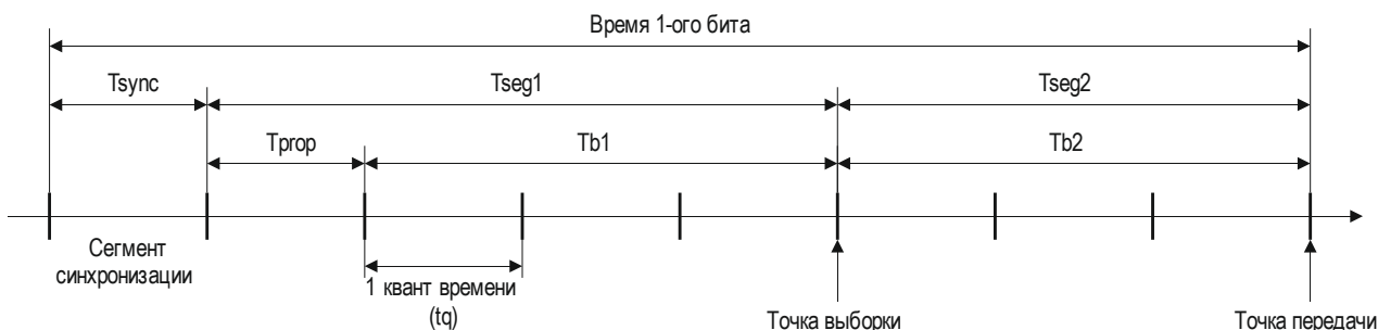
Рисунок 18.14 – Структура одного бита
