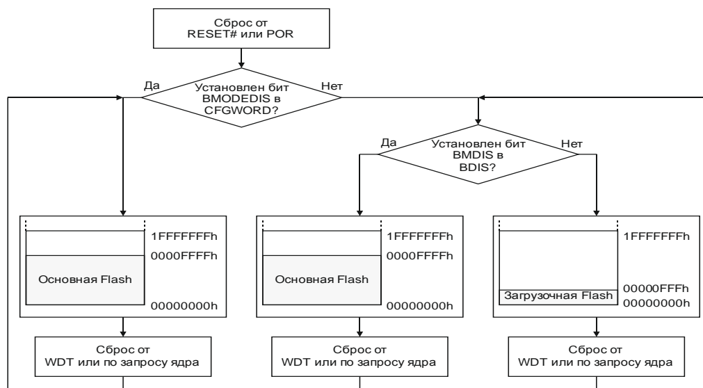
Рисунок 7.1 – Блок-схема алгоритма загрузки микроконтроллера
