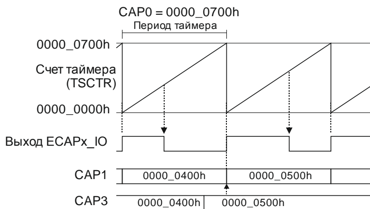
Рисунок 12.4 – Пример формирования сигнала ШИМ с активным высоким уровнем сигнала (по умолчанию APWMPOL = 0 )
