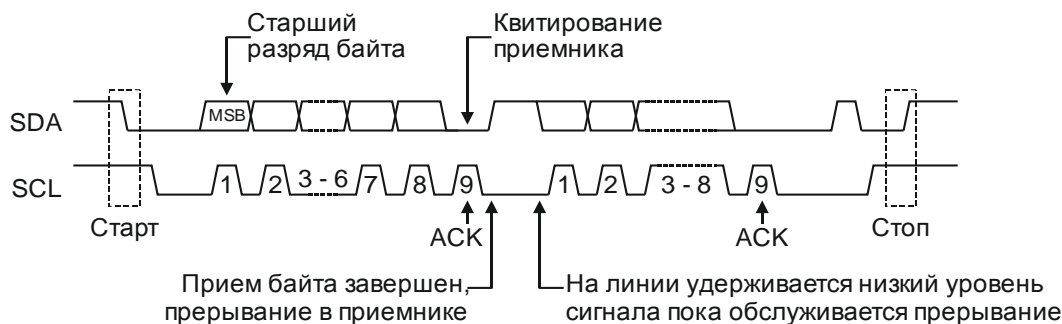
Рисунок 17.6 – Передача данных
