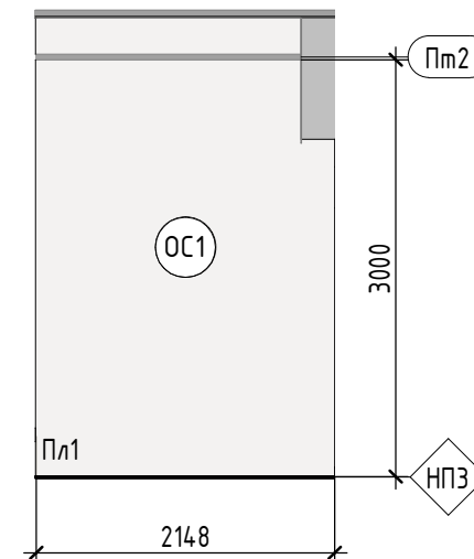
1018.6 (1 : 60)
