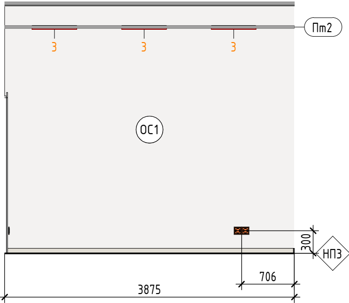
1028.2 ( 1 : 50)
