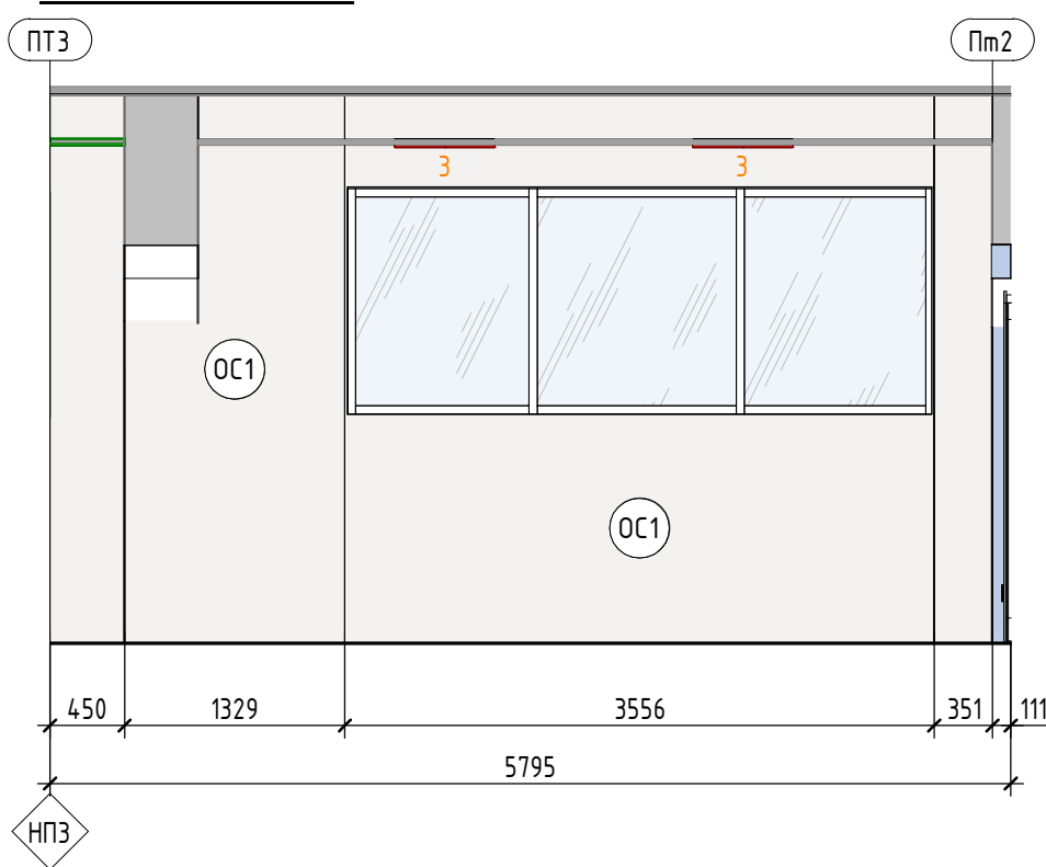
Кабинет 103а.3 ( 1 : 50)
