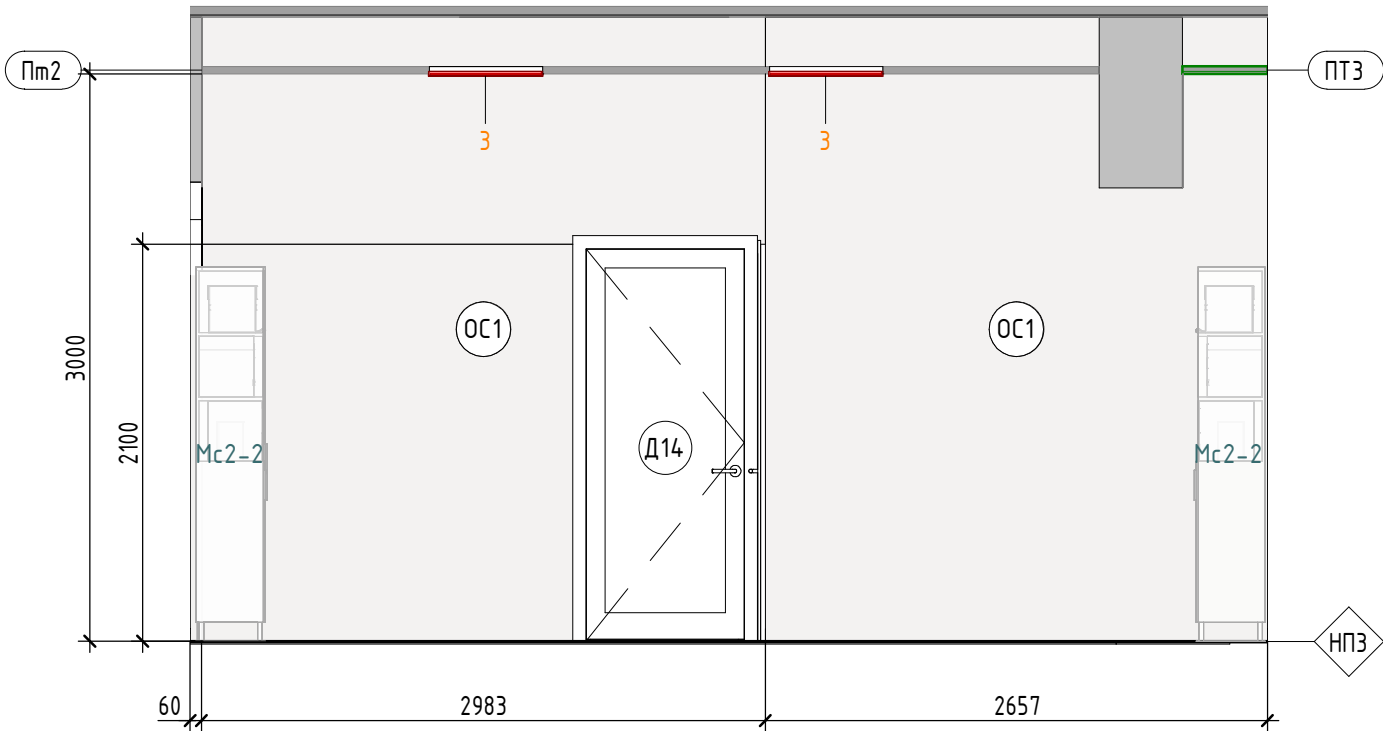
Кабинет 1038 (1 : 130)
