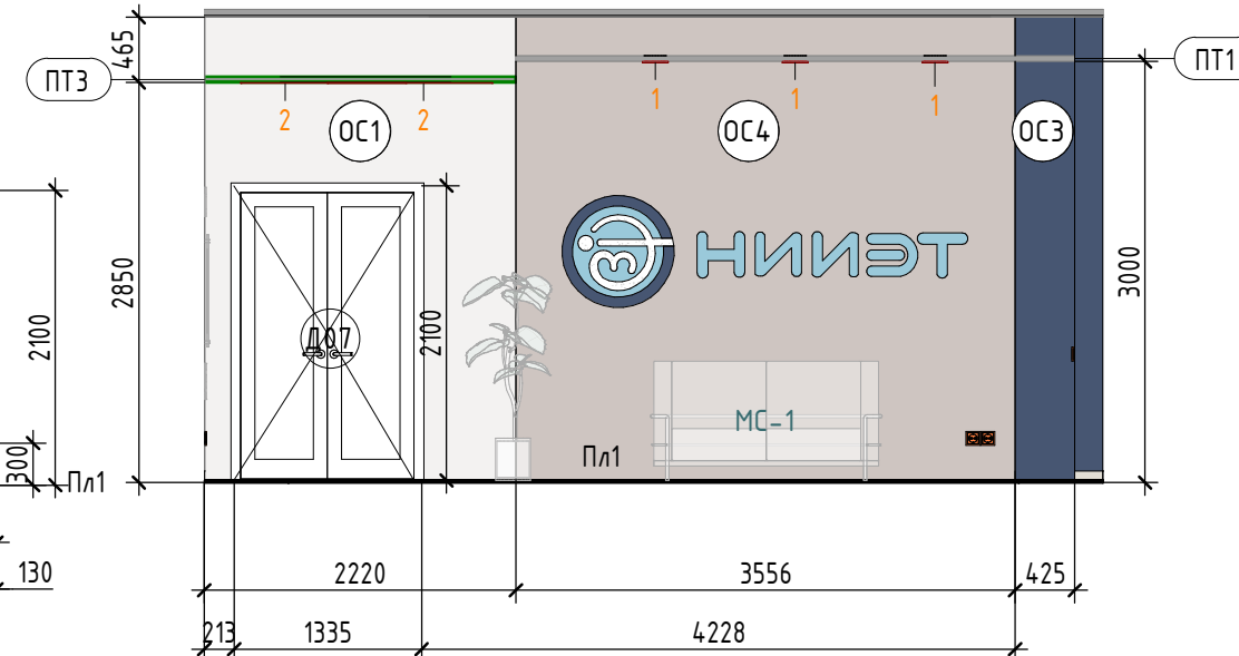
фойе5 (1: 60)
