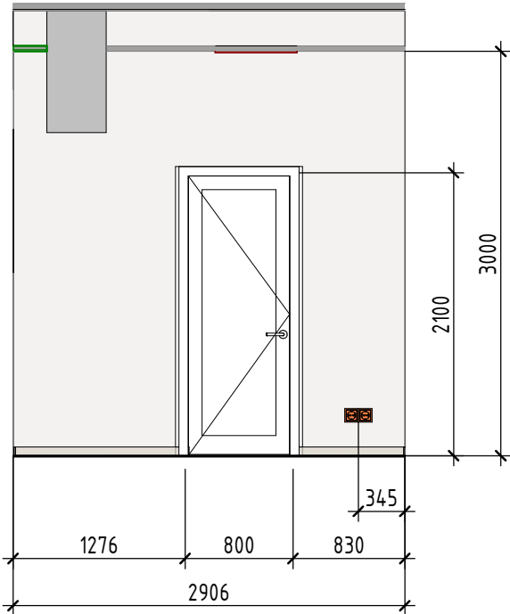
1028.3 ( 1 : 50)
