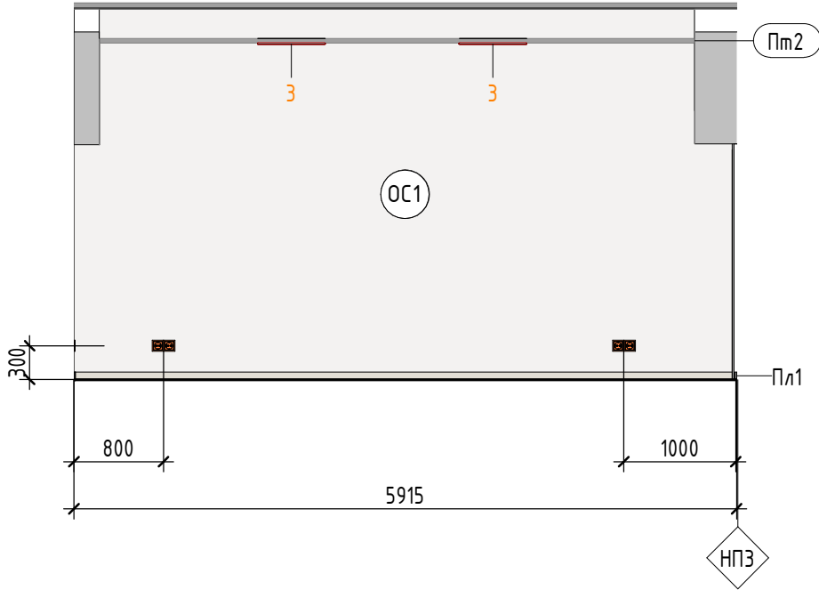
101а.3 (1 : 60)
