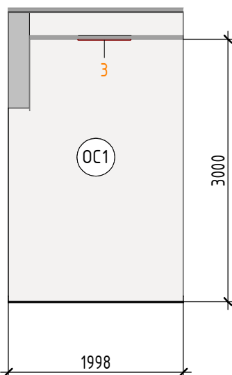
101z.3 (1 : 60)
