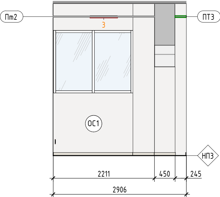
1028.1 ( 1 : 50)
