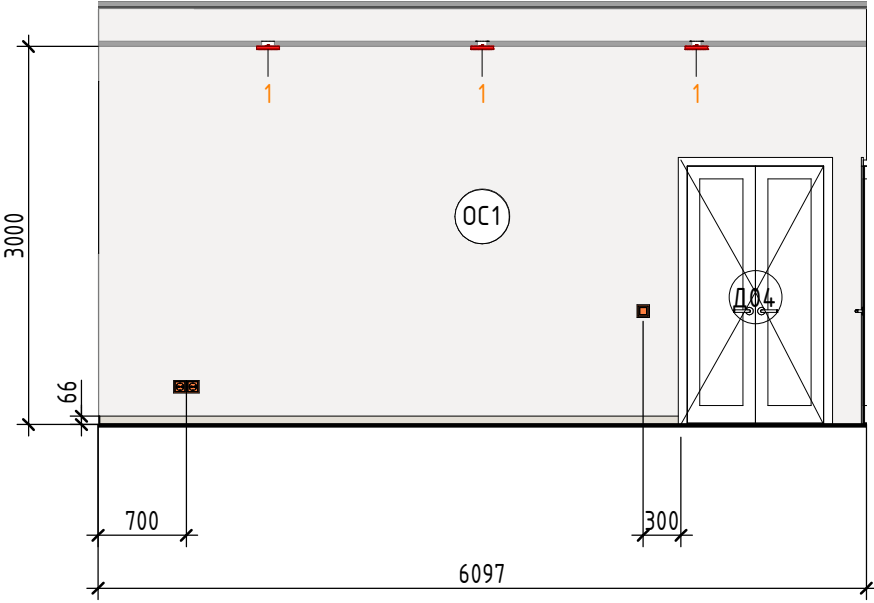
101б.4 (1 : 60)
