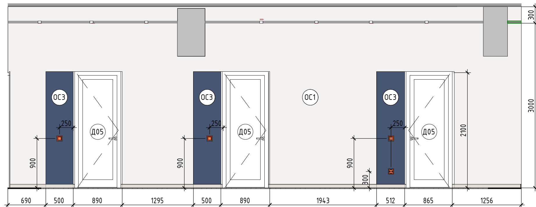
кор2.6 (1 : 40)
