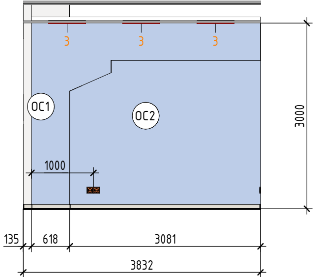
101а.4 (1 : 60)
