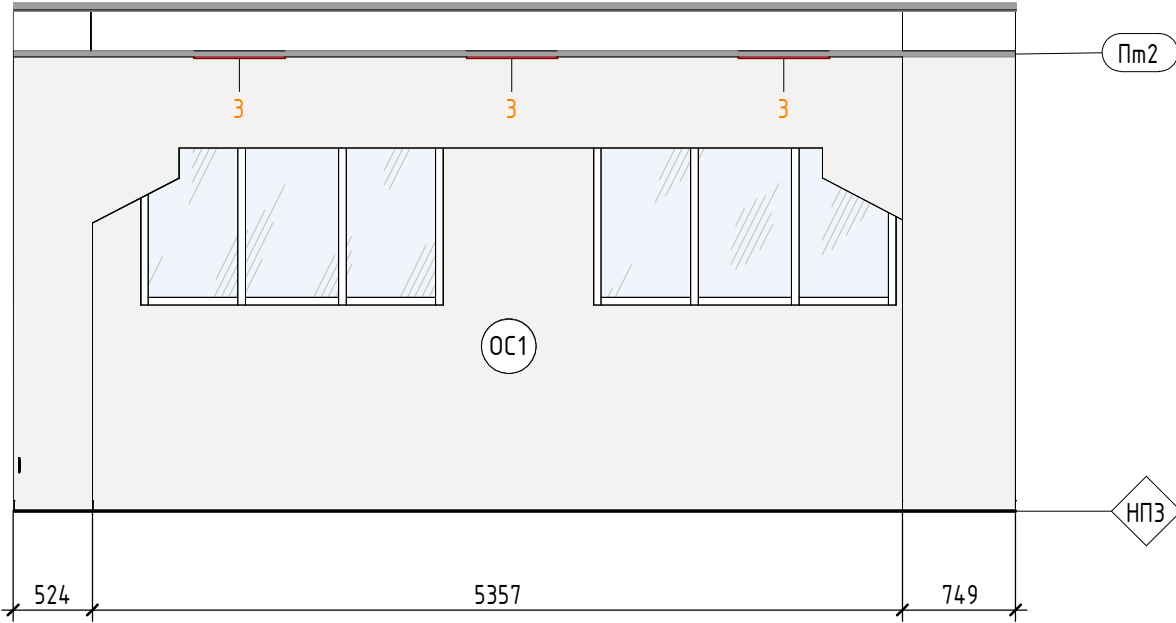
Кабинет 103а.2 ( 1 : 50)
