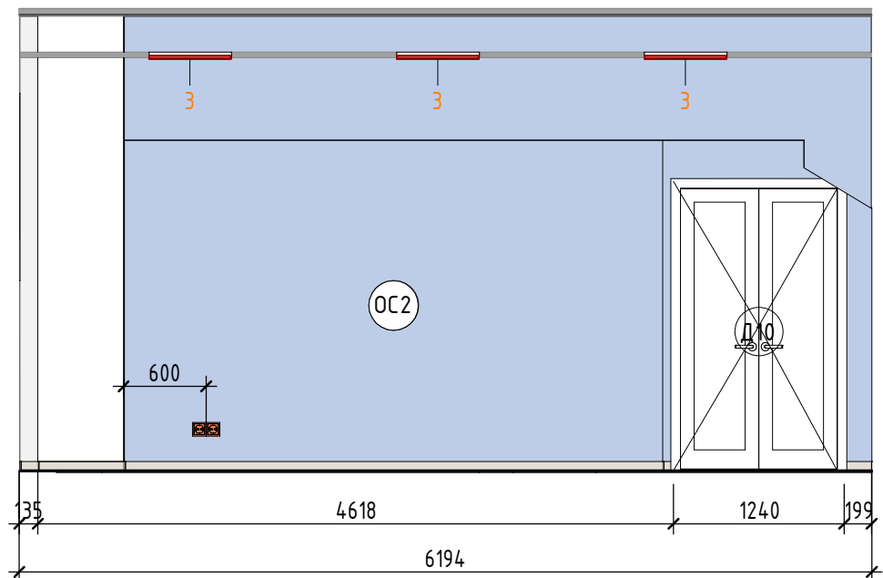
Кабинет 103 ( 1 : 100)
