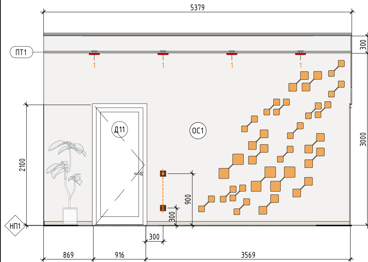
кор2.1 (1 : 40)
