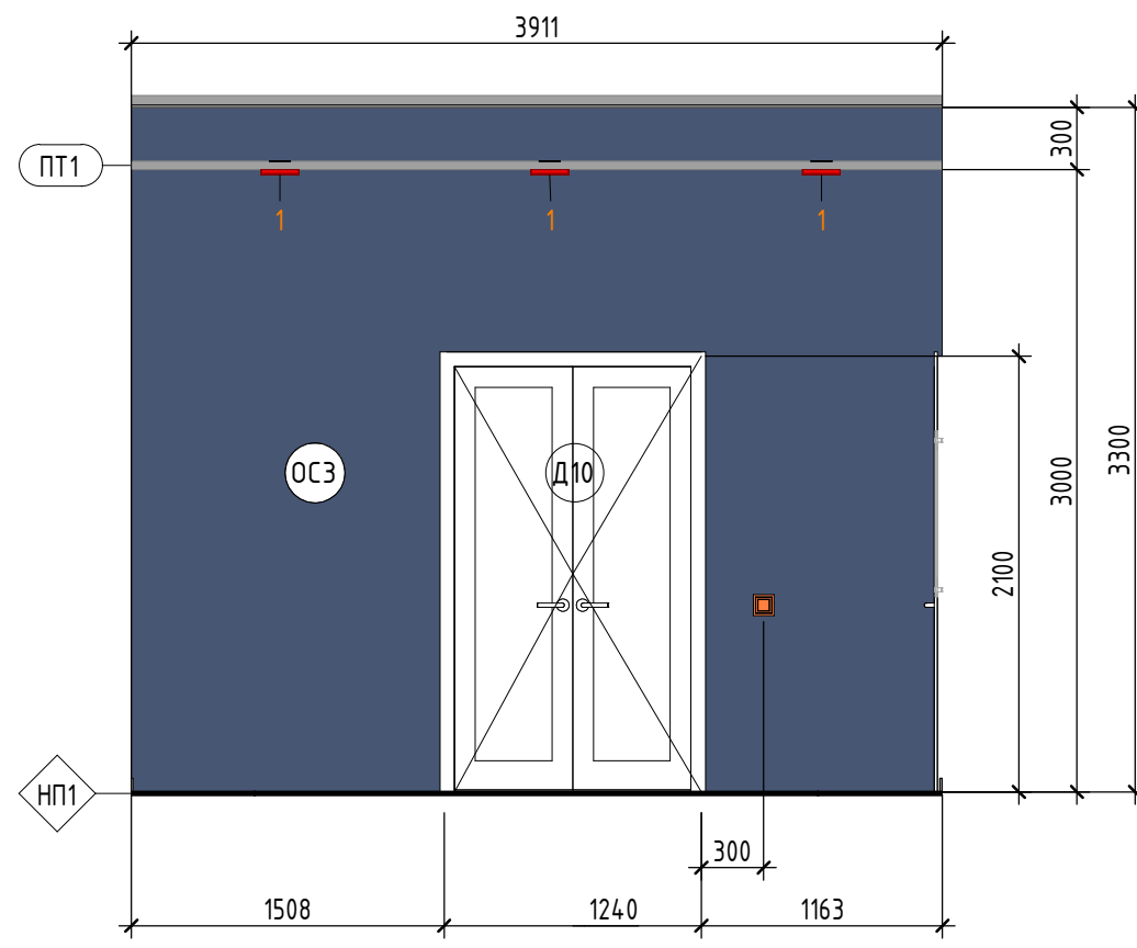
кор2.2 (1 : 40)
