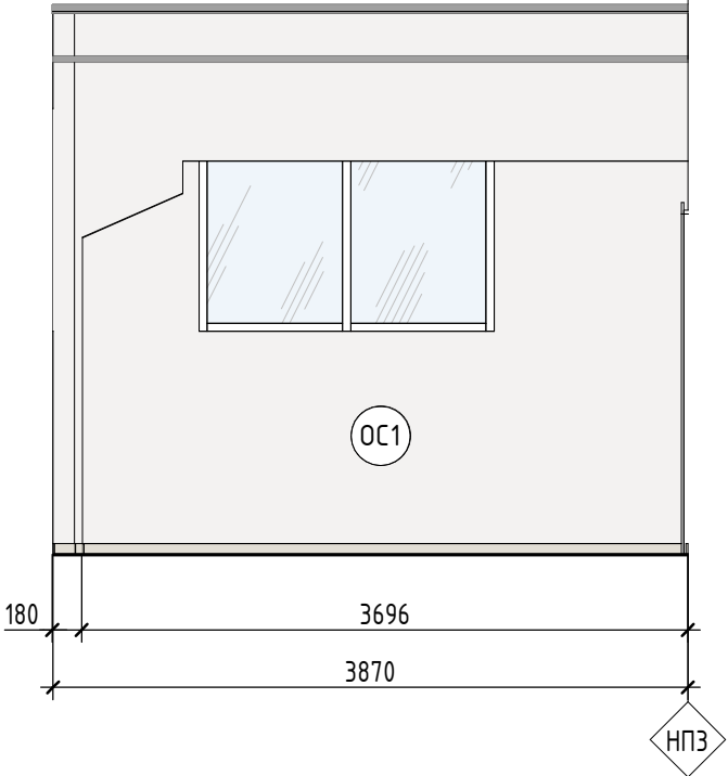
1028.2 ( 1 : 50)
