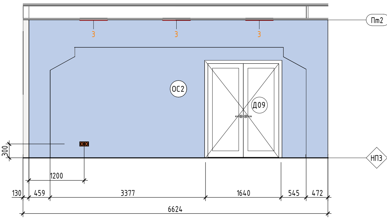
Кабинет 103а.4 ( 1 : 50)
