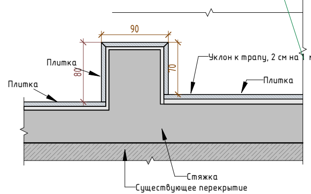
Порог душевой ( 1 : 5 )
