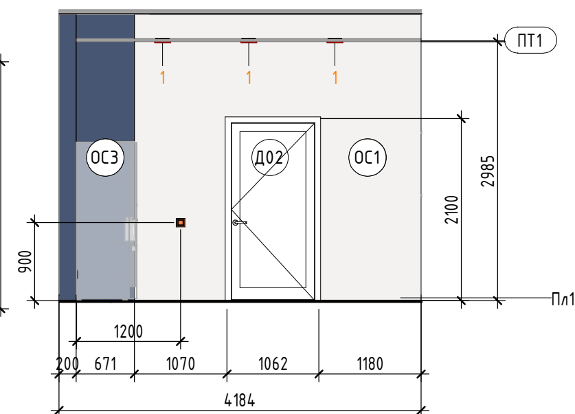
фойе4 (1: 60)
