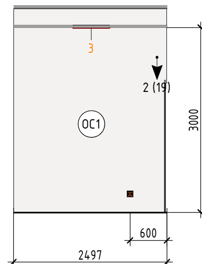
101z.4 (1 : 60)
