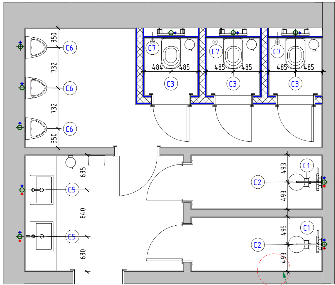
Фр.2 (1 : 40)
