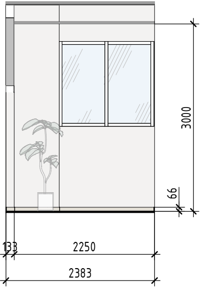
101а.4 (1 : 60)
