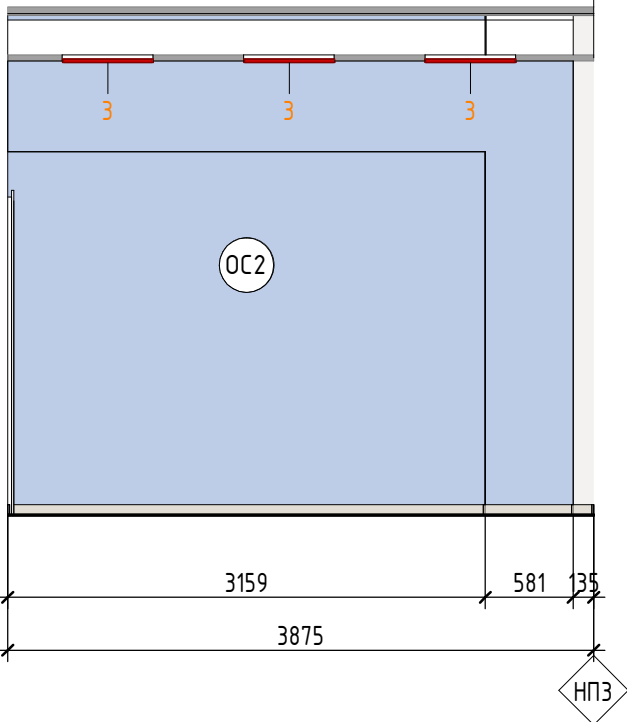
1028.3 ( 1 : 50)
