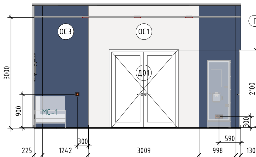
фойе2 (1: 60)
