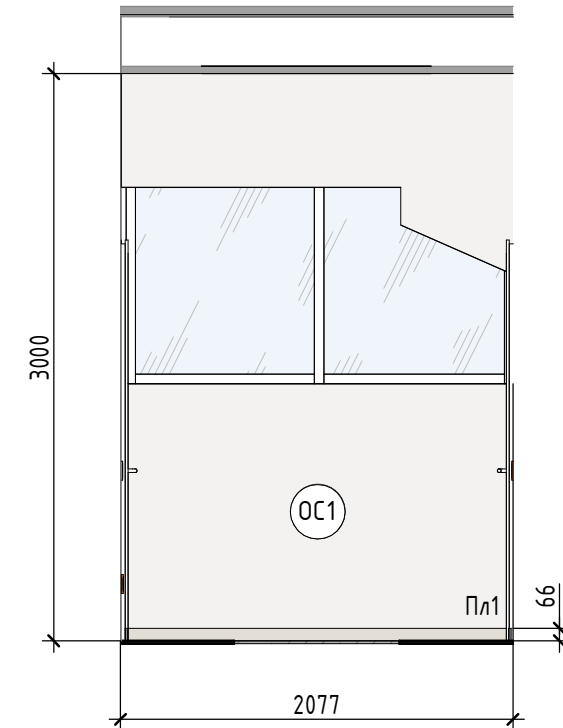
кор 2.4 (1 : 40)
