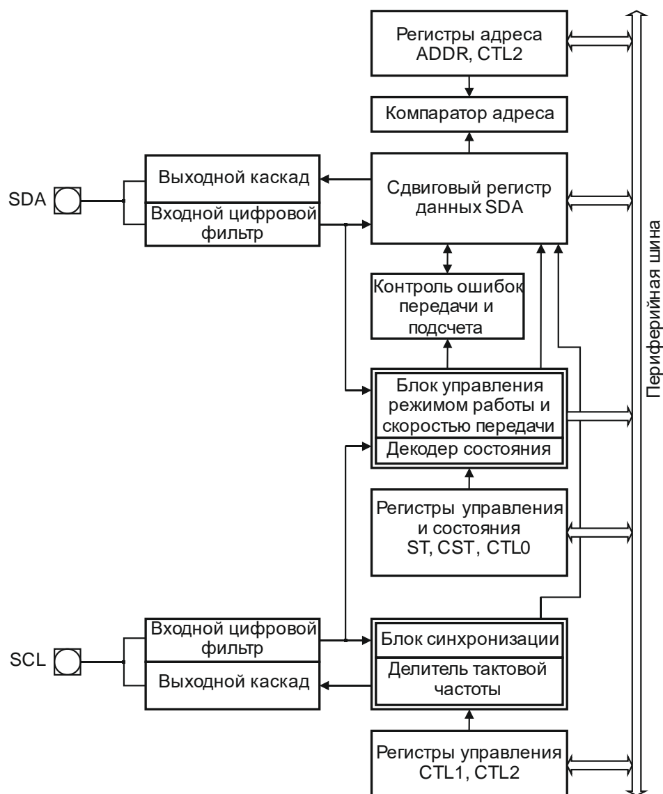
Рисунок 17.12 – Структурная схема модуля I2C
