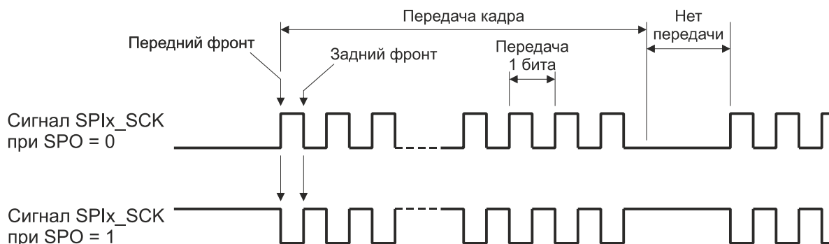
Рисунок 16.2 – Сигнал синхронизации SPI_SCK при разных состояниях бита SPO
