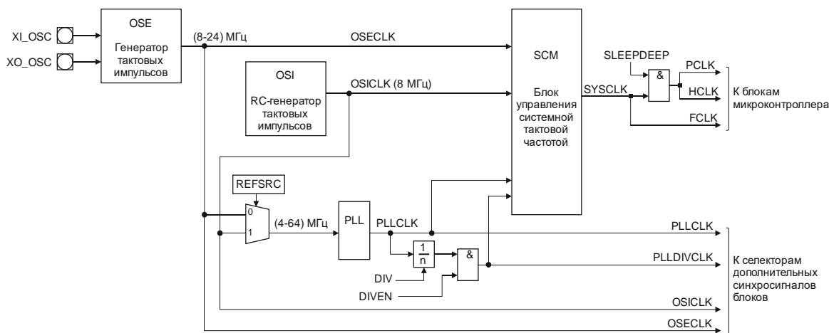
Рисунок 4.1 – Схема синхронизации
