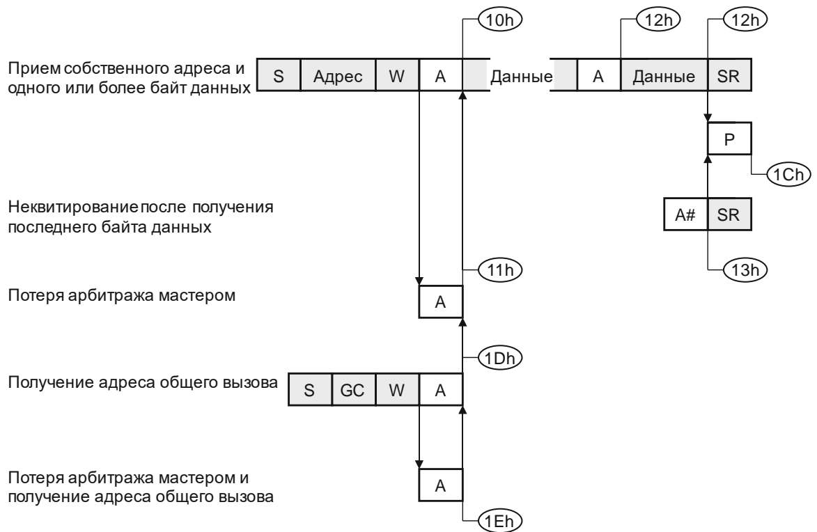
Рисунок 17.20 – Режим FS ведомого приемника
