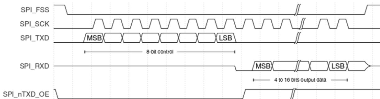
Рисунок 16.5 – Передача кадра данных в интерфейсе Microwire
