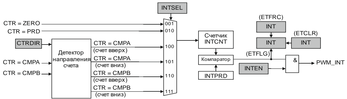
Рисунок 14.20 – Функциональная схема триггера событий для генерации прерываний
