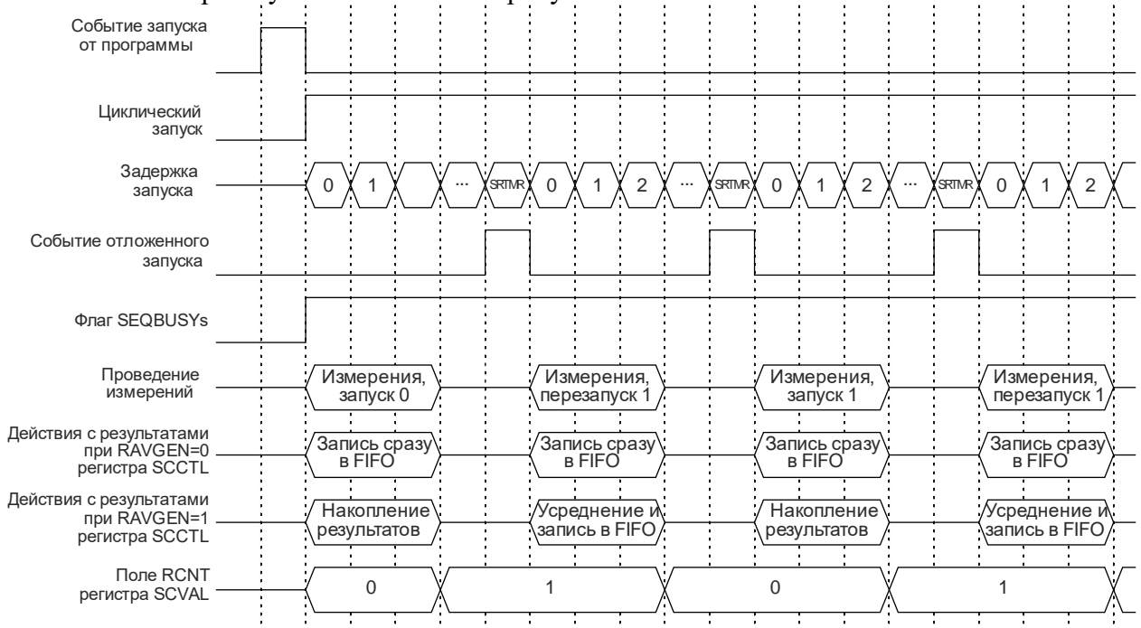
Рисунок 19.9 – Диаграммы работы секвенсора в циклическом режиме запуска с усреднением по отложенным перезапускам определённое время (значение регистра SRTMR) при RCNT=1 (регрстр SCCTL)
