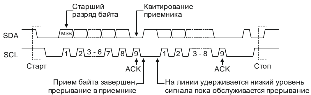
Рисунок 17.6 – Передача данных
