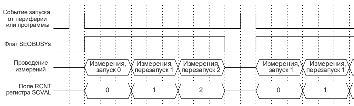
Рисунок 19.4. – Одиночные запуски по событиям с немедленными перезапусками при RCNT = 2 (регистр SCCTL)
