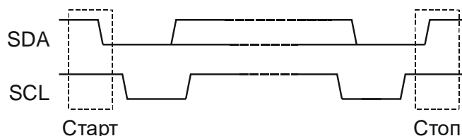
Рисунок 17.2 – Состояния старта и стопа
