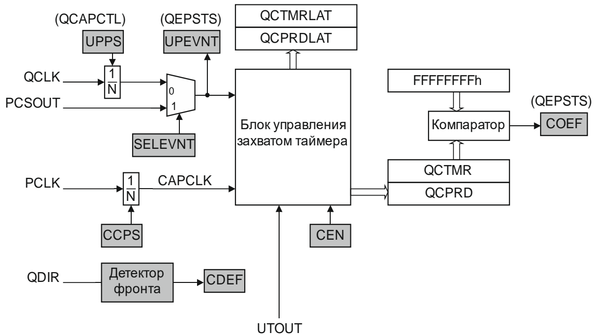
Рисунок 13.9 – Функциональная схема модуля захвата времени
