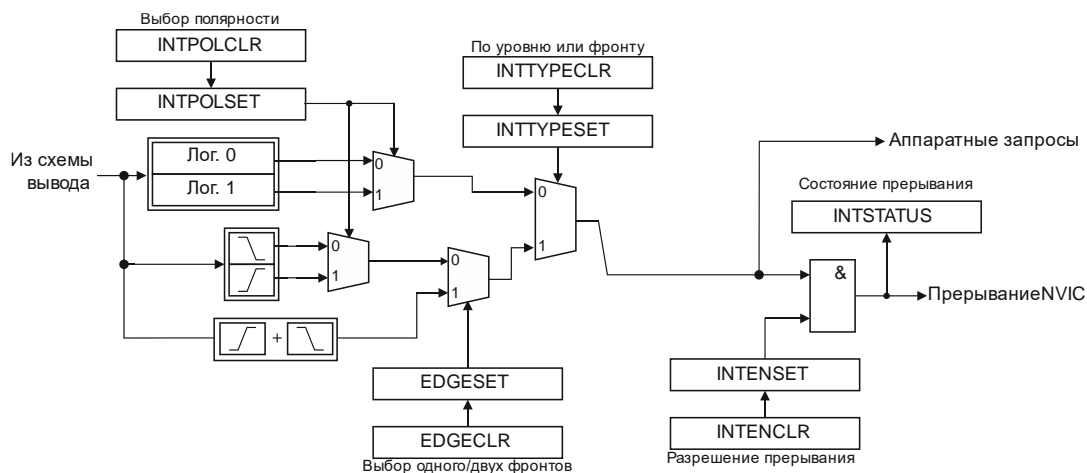
Рисунок 10.3 – Структурная схема блока генерации прерываний
